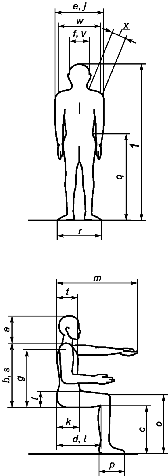
Рисунок Д.1 — Размеры тела пассажиров
