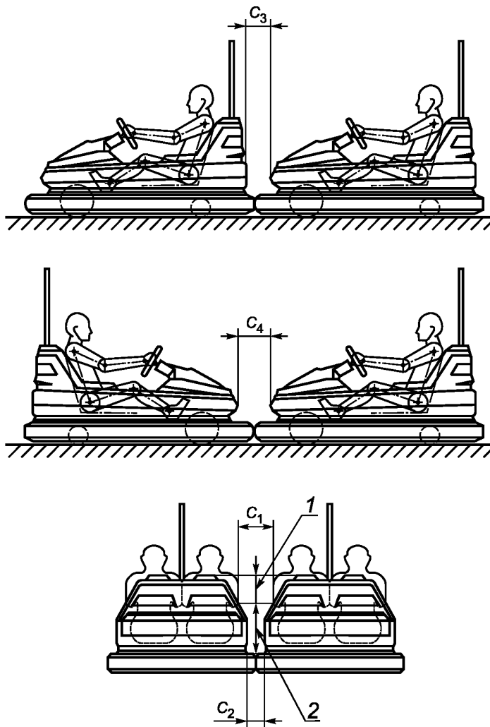
Рисунок 15 — Сталкивающиеся автомобили, лист 1
