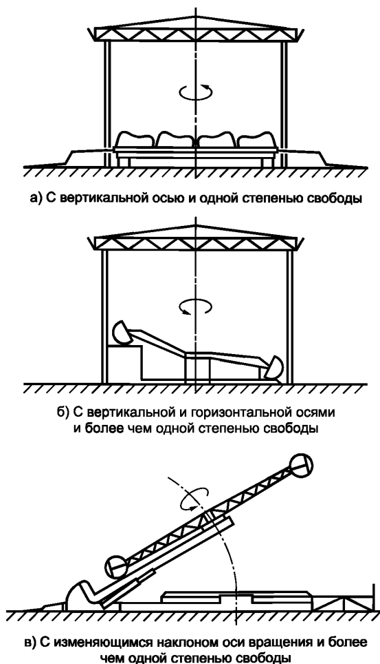
Рисунок 12 — Карусели с вертикальным и/или горизонтальным движением, лист 1
