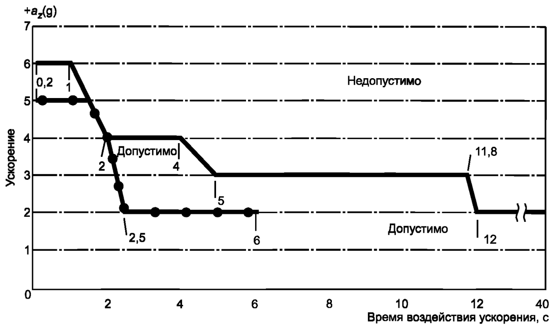
Рисунок А.2 — Длительность предельно допустимых линейных ускорений «таз — голова» a_z(g)_{max} для пассажира аттракциона, зафиксированного в кресле в позе «сидя», при единичном воздействии импульса
