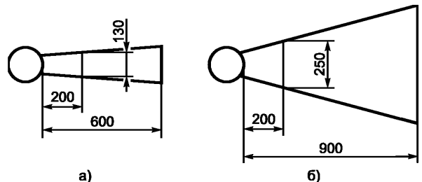
Рисунок 2 — Размеры спиральных и винтовых лестниц
