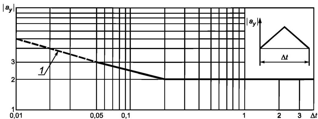
Рисунок Б.1 — Допустимое ускорение сиденья |a_y| в зависимости от длительности импульса
