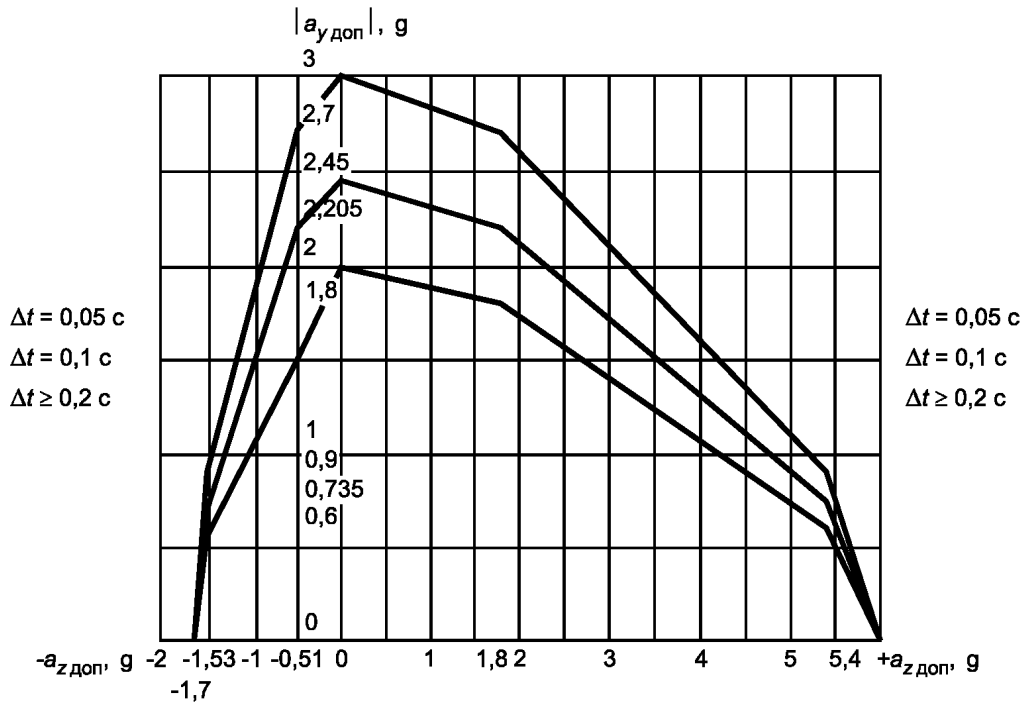
Рисунок Б.4 — Допустимые ускорения a_y и a_z при их совместном воздействии
