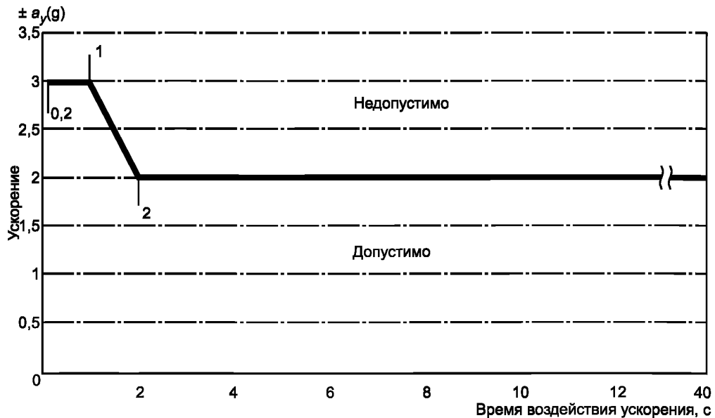
Рисунок А.6 — Длительность предельно допустимых линейных ускорений «бок — бок» \pm a_y(g) для пассажира аттракциона, зафиксированного в кресле в позе «сидя» или «лежа», при единичном воздействии импульса
