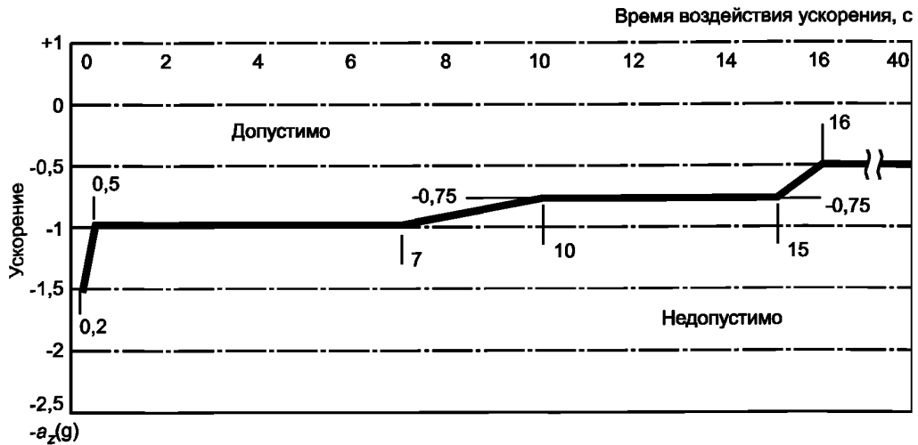
Рисунок А.3 – Длительность предельно допустимых линейных ускорений «голова — таз» -a_z(g) для пассажира аттракциона, зафиксированного в кресле в позе «сидя», при единичном воздействии импульса
