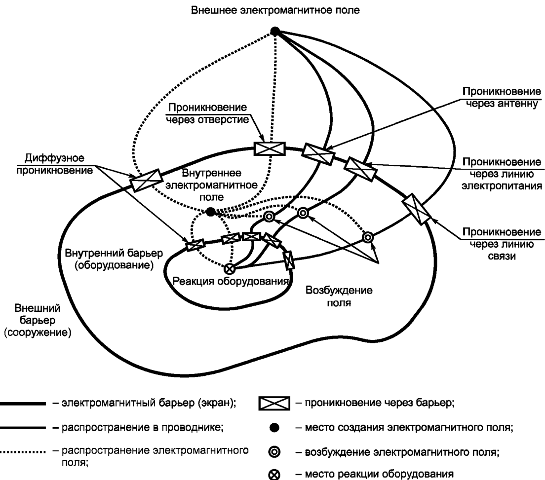
Рисунок 6 — Топологическая схема простой системы, представленной на рисунке 5
