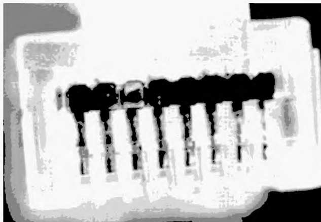
Рисунок 9 — Пример повреждений, вызванных одиночным импульсом напряжением 4,5 кВ испытательного генератора МИП ( 6,5/700 мкс — 4/300 мкс) по ГОСТ Р 51317.4.5
