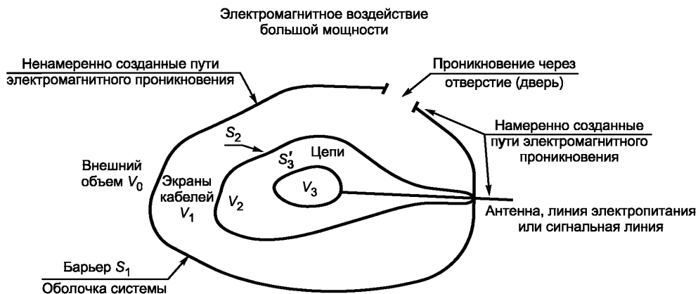
Рисунок 11 — Схема намеренно и ненамеренно созданных путей электромагнитного проникновения применительно к системе, представленной на рисунке 5
