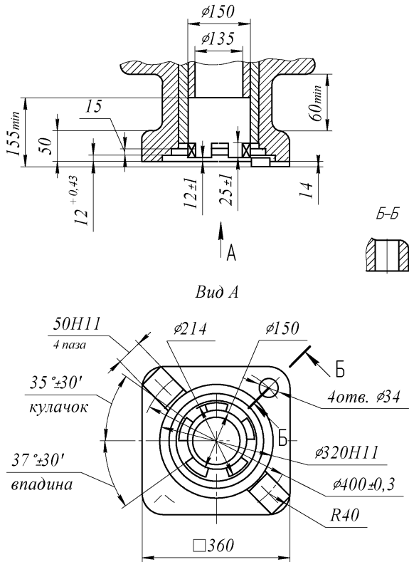
Рисунок А.13 – Присоединение привода типа Д
