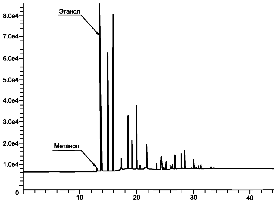
Рисунок 1 — Пример хроматограммы
