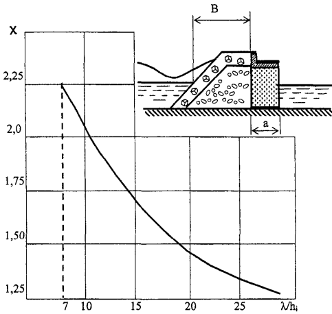
Рисунок 5.8 - График для определения коэффициента X = f(\bar{\lambda}/h)
