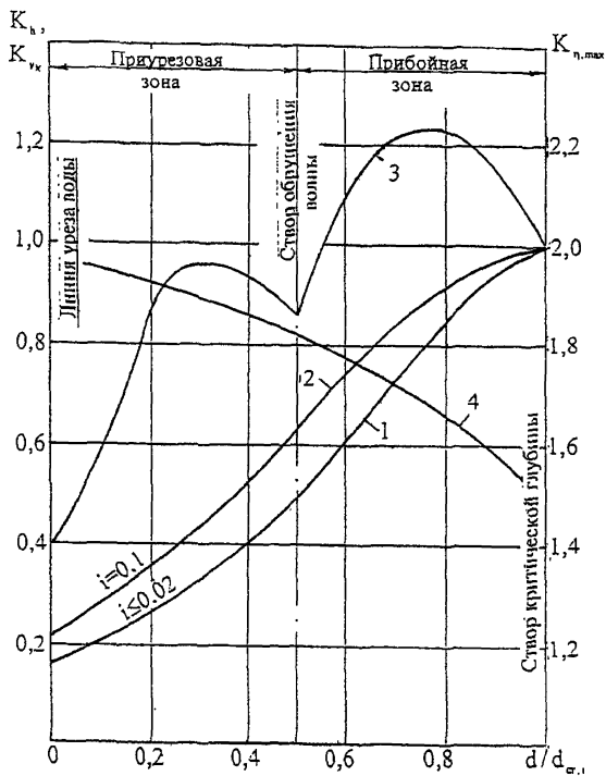
Рисунок А.3 - Графики для определения коэффициентов K_k (1 и 2), K_{v,k} (3) и K_{n,max} (4)
