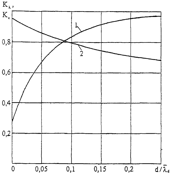
Рисунок А.2 - Графики для определения коэффициентов K_\lambda (1) и K_\epsilon (2)
