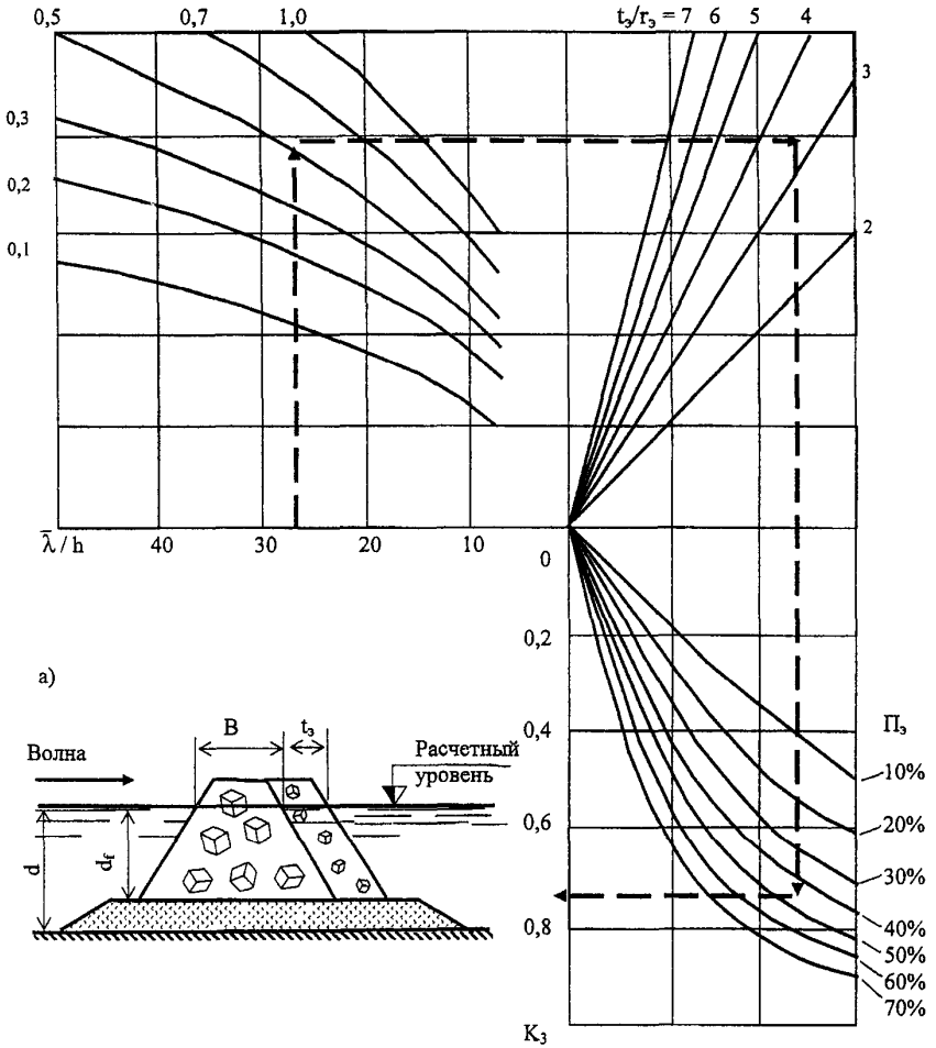
Рисунок 5.7 - Схема (а) и графики (б) для определения коэффициента загухания волн K_3 при наличии тылового экрана в набросном сооружении
