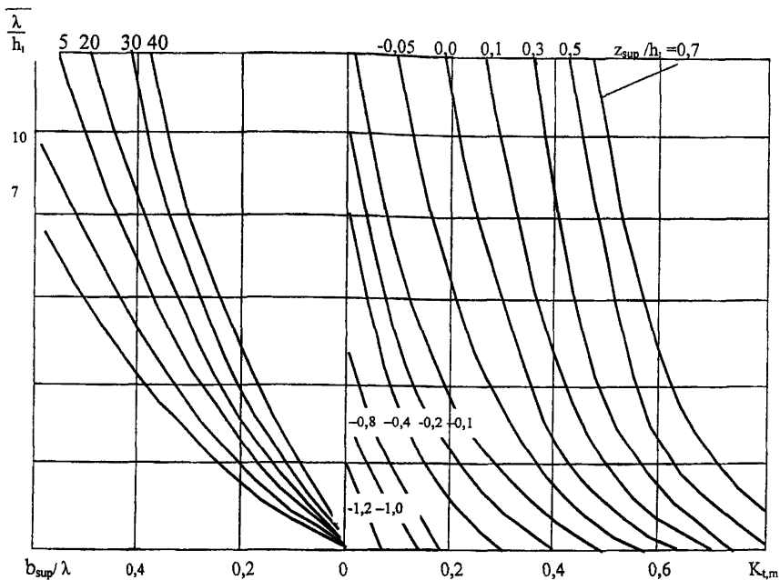
Рисунок 5.5 - Схема (а) и графики (б) для определения коэффициентов прохождения K_{t,m} ветровых волн через верх набросного сооружения неполного профиля с ядром из несортированного камня
