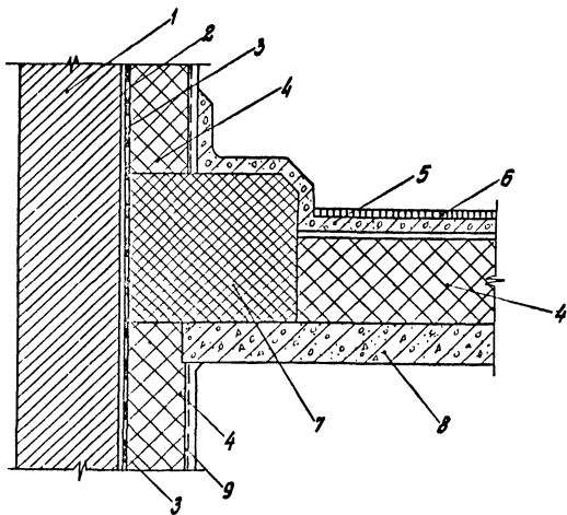
Рис. 5.1. Притыкание междуэтажных перекрытий к наружным стенам. 1- наружный (несущий) слой; 2- штукатурка (при кирпичных и блочных стенах); 3- негорючий паразитизирующий слой; 4- теплоизоляционный слой; 5- армированная бетонная стяжка; 6- пол; 7- противопожарный пояс; 8- междуэтажное перекрытие; 9- отделочный слой.
