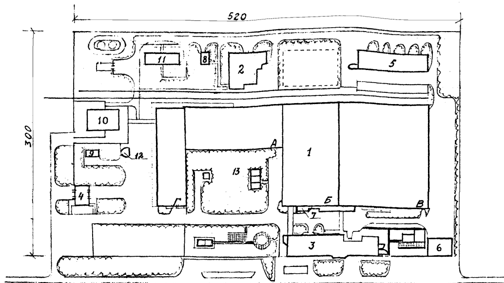
Рис. 2.4. Типовое проектное решение мяскокомбината мощностью 100 тонн мяса в смену. 1- главное производственное здание: А- мясожировой корпус, Б- холодильник, машинное отделение и трансформаторная подстанция, В- мясоперерабатывающий корпус, Г- корпус предубойного содержания скота; 2- корпус технических фабрикатов; 3- административно-бытовой корпус; 4- пункт мойки и дезинфекции автомашин; 5- блок подсобных цехов; 6- весовая с 15 и 30т весами; 7- конденсаторная установка; 8- песколовка-жироловка; 9- дезинфектор; 10- санитарный блок; 11- котельная; 12-каньная на 3 пресса; 13- вентиляторная градирня.
