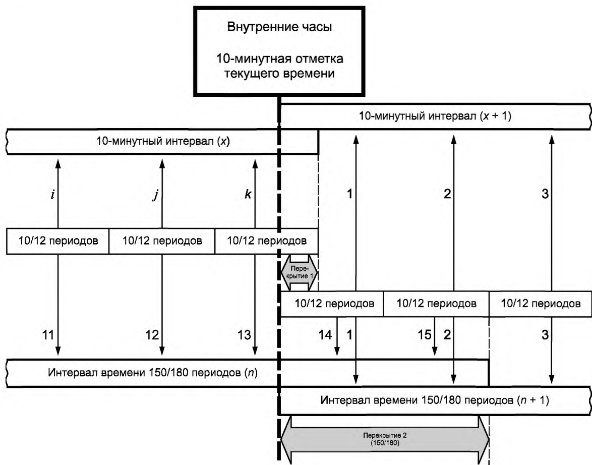
Рисунок 2 — Синхронизация объединенных интервалов для класса А
