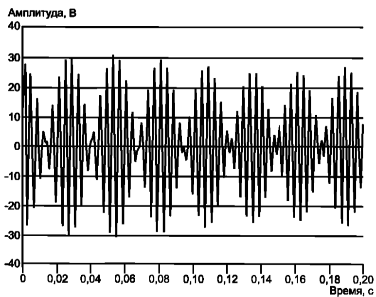
е) Сумма гармоники и интергармоники
