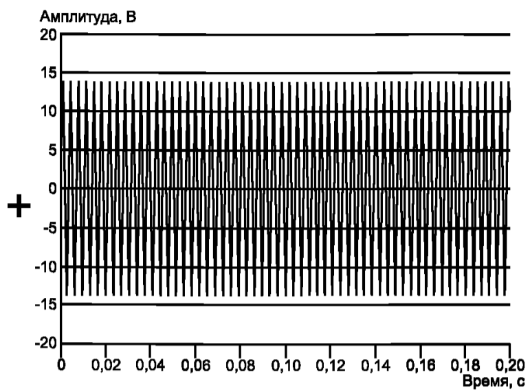
б) Интергармоника 287 Гц
