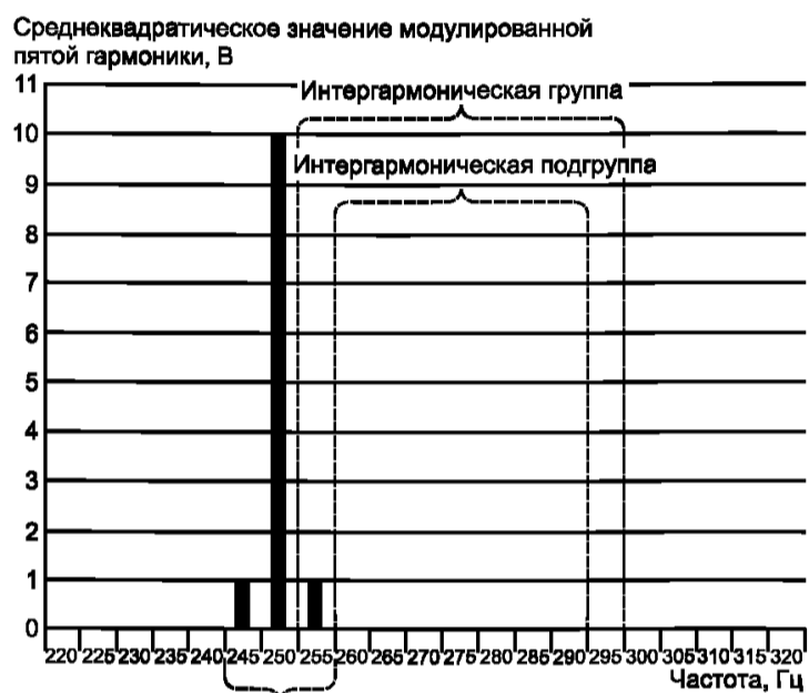
с) Спектр пятой гармоники с 20 %- ной амплитудной модуляцией
