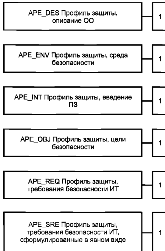
Рисунок 6 — Декомпозиция класса APE «Оценка профиля защиты»
