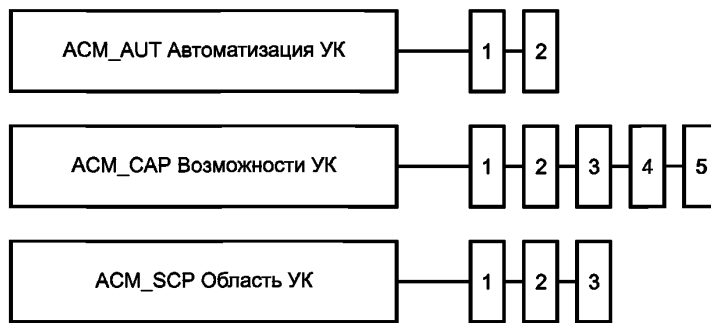
Рисунок 8 — Декомпозиция класса ACM «Управление конфигурацией»
