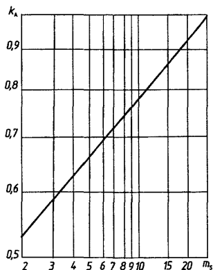
Рис. 2. Определение коэффициента k_A
