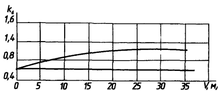
Рис. 3. Определение коэффициента k_d
