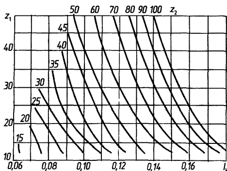
Рис. 4. График для определения коэффициента I_k при расчете на контактную выносливость ( \alpha_{\text{ср}} = 20^\circ ; \beta_{\text{ср}} = 35^\circ )
