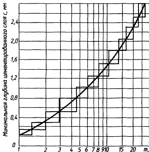
Рис. 5. График для определения минимальной глубины цементированного слоя
