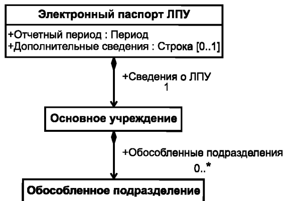
Рисунок А.3 — Данные о ЛПУ
