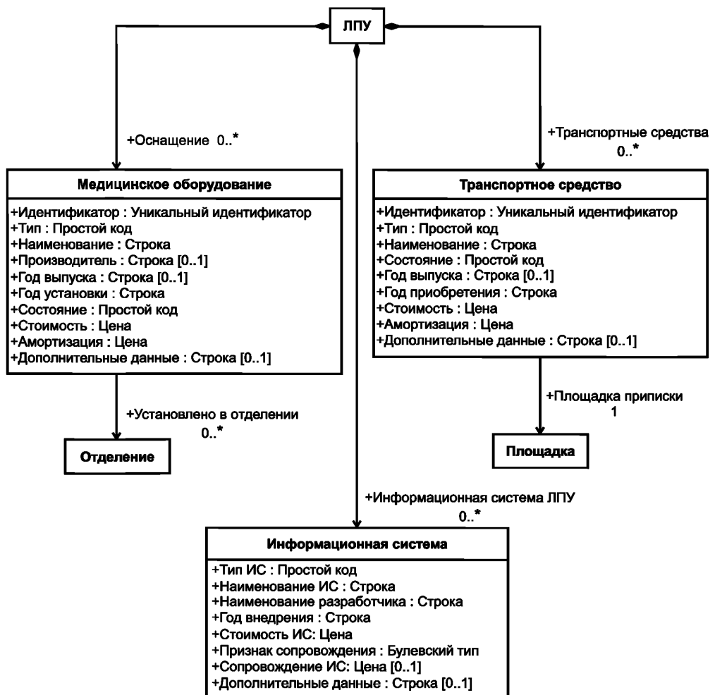
Рисунок А.6 — Оснащение ЛПУ
