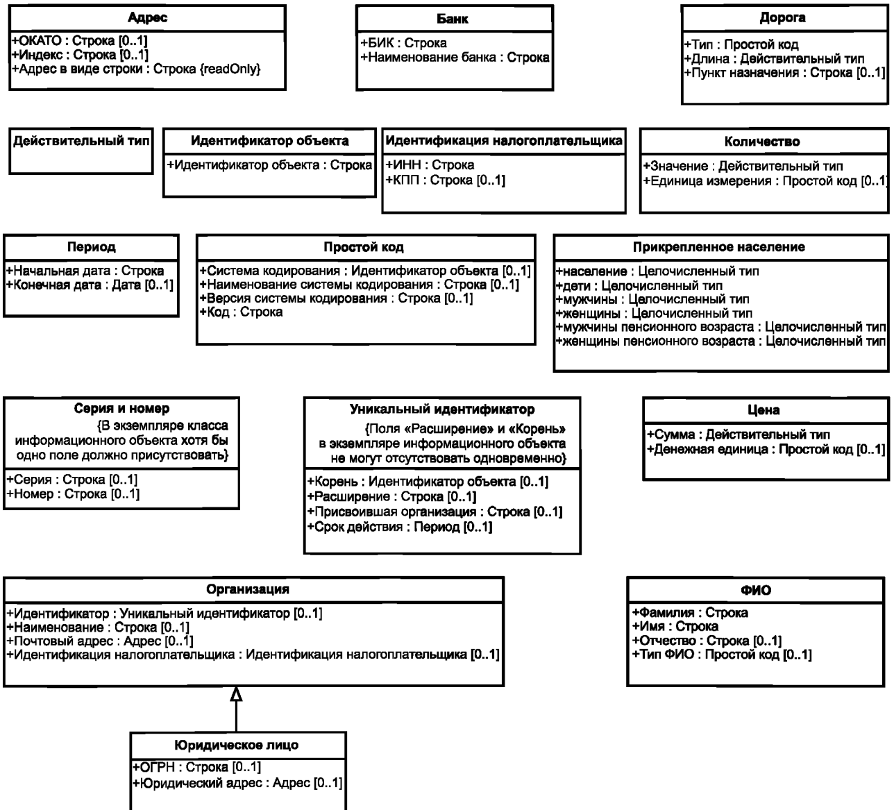
Рисунок А.2 — Вспомогательные классы
