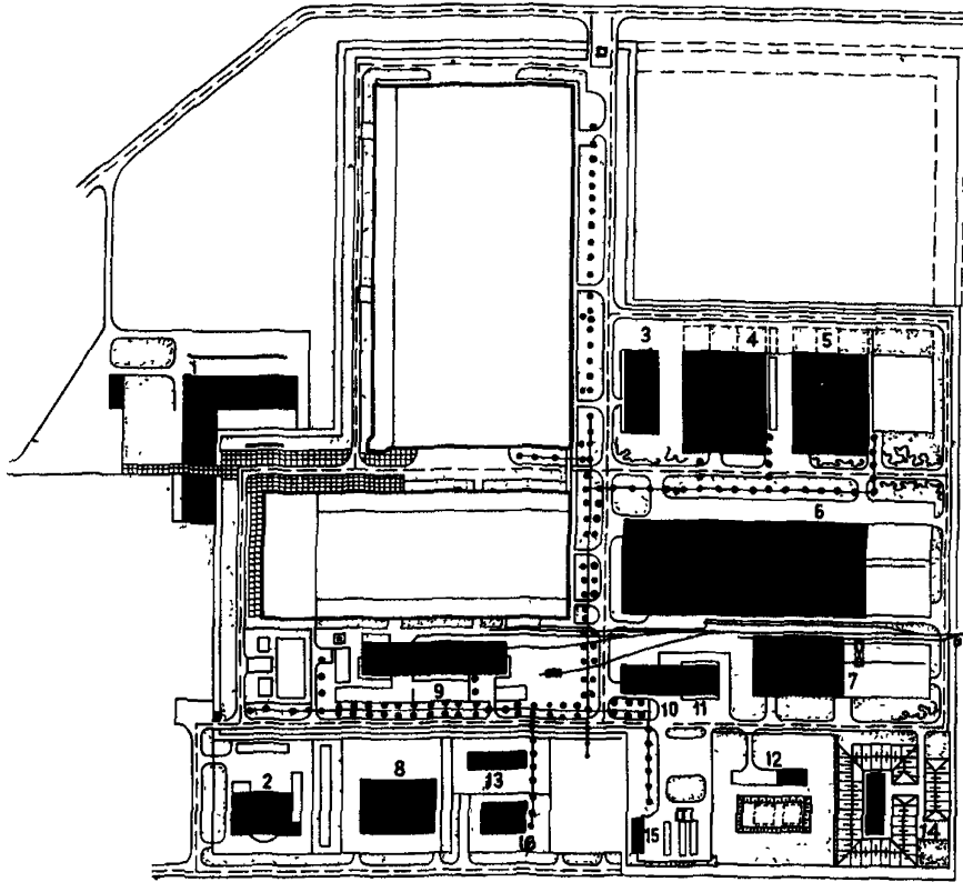
Рис. 9. Проект генерального плана предприятия химического волокна 1 — заводоуправление; 2 — корпус спасательных служб; 3 — лабораторный корпус; 4 — корпус обще заводских энергетических служб; 5 — корпус химической очистки воды; 6 — объединенный корпус ремонтно-складских служб; 7 — склад тяжеловесов; 8 — пункт технического обслуживания уборочных и спецмашин; 9 — объединенный склад жидких и газообразных продуктов; 10 — склад масел, красок, химикатов; 11 — прачечная спецодежды; 12 — насосная станция водного хозяйства; 13 — цех наполнения и хранения баллонов; 14 — склад порофора; 15 — объединенная канализационная насосная станция; 16 — тепловой пункт
