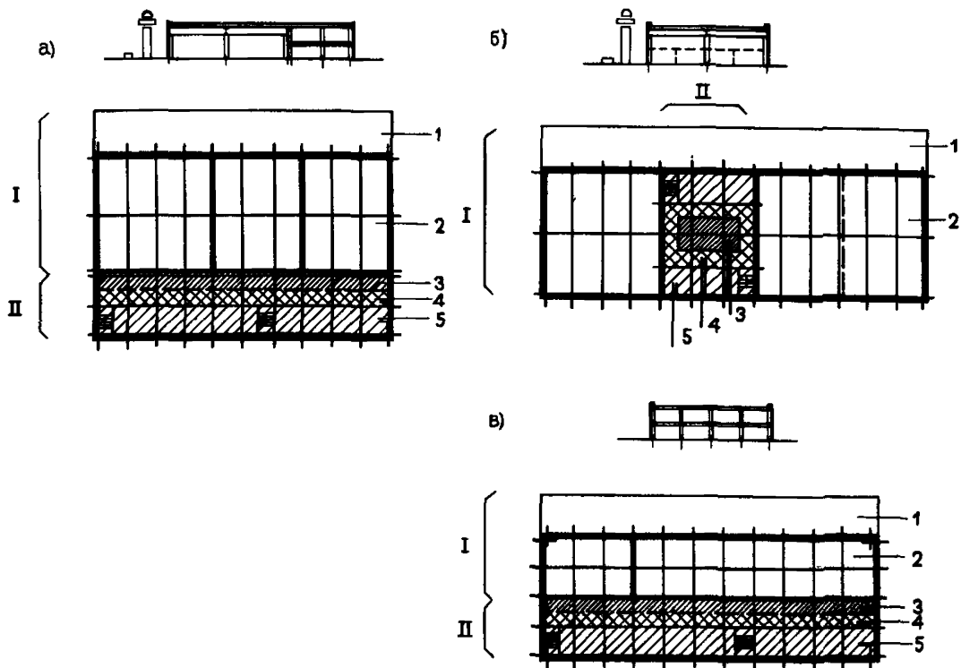
Рис. 17. Варианты объемно-планировочного решения блокированных зданий а, б — одноэтажные здания с протяженным и концентрированным размещением блока "обеспечения"; в — многоэтажные здания; 1 — технологические блоки; II — блоки "обеспечения"; 1 — открытая площадка для оборудования или хозяйственный двор; 2 — производственные помещения; 3 — "темная" зона; 4 — транзитный коридор; 5 — "светлая" зона
