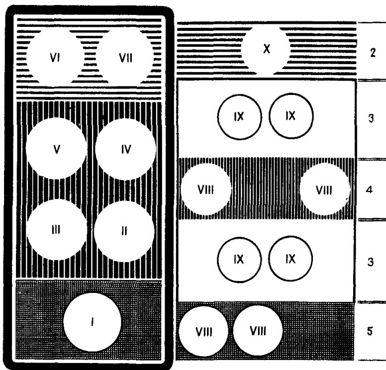
Рис. 5. Функциональные группы объектов I – объекты предзаводской площадки; II – объекты общезаводских подсобных и хозяйственных служб; III – объекты водного хозяйства; IV – объекты общезаводских энергетических служб; V – объекты общезаводских ремонтных служб; VI – общезаводские склады; VII – объекты железнодорожного транспорта; VIII – межпроизводственные подсобные и вспомогательные объекты; IX – межцеховые подсобные и вспомогательные объекты; X – склады сырья и готовой продукции; 1 – общезаводские объекты; 2 – складская зона; 3 – производственная зона; 4 – зона подсобных объектов; 5 – предзаводская зона
