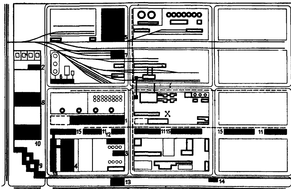
Рис. 6. Проект генерального плана предприятия азотных удобрений 1 — корпус энергетических служб; 2 — насосная станция водного хозяйства; 3 — корпус азото-и воздуходооборудования; 4 — корпус ремонтных служб; 5 — склады оборудования и материалов; 6 — насосная станция склада жидких и газообразных продуктов; 7 — корпус железнодорожного транспорта; 8 — гараж саноборочных и спецмашин; 9 — комплекс управления предприятием; 10 — цех подсобного хозяйства; 11 — корпус межпроизводственных энергослужб; 12 — канализационная насосная станция; 13 — главная понизительная подстанция; 14 — входной блок; 15 — административно-бытовой блок
