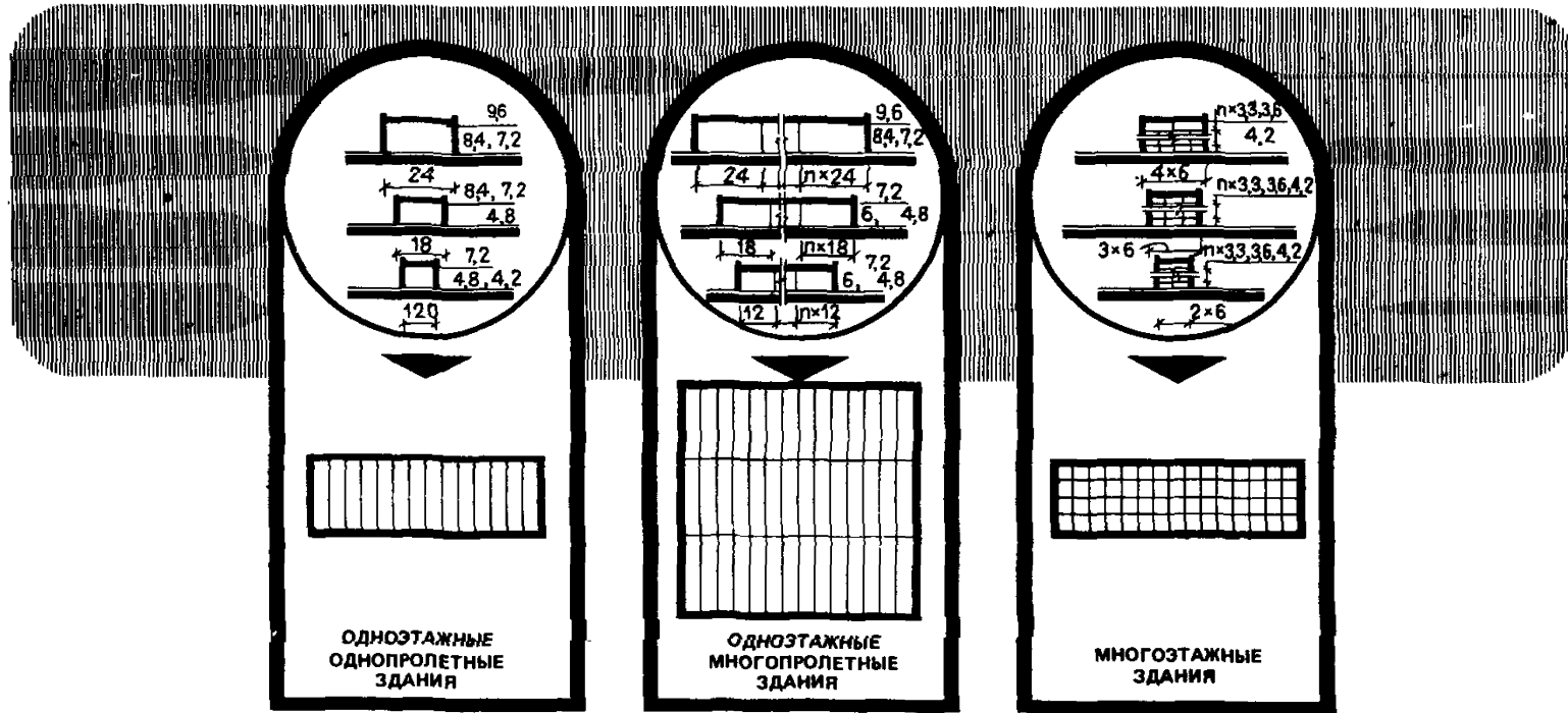
Рис. 11. Унификация габаритных схем объектов
