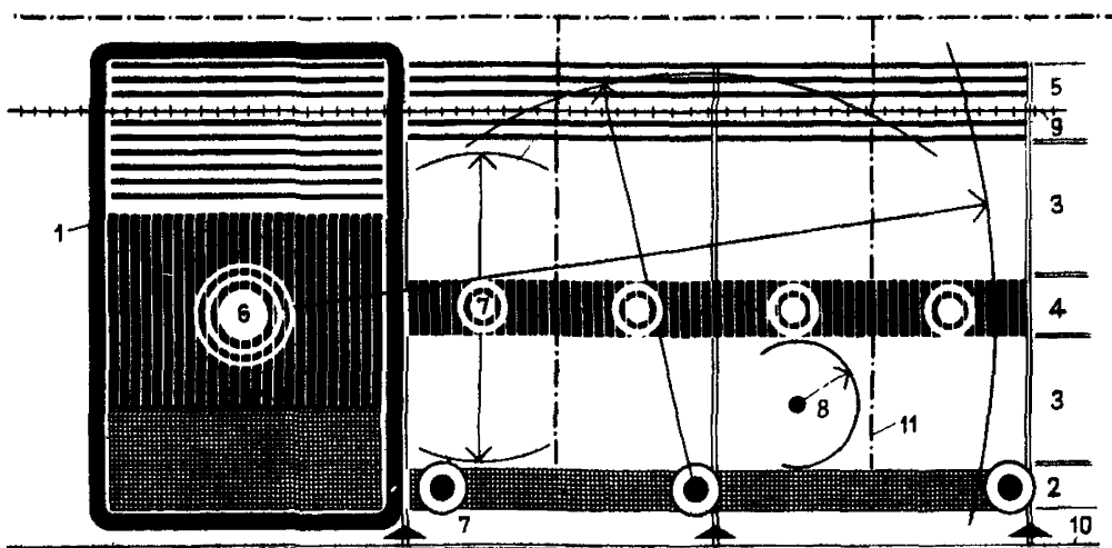
Рис. 3. Структурно-функциональная модель размещения объектов 1 — зона общезаводских объектов; 2 — предзаводская зона; 3 — производственная зона; 4 — подсобная зона; 5 — складская зона; 6 — общезаводские объекты; 7 — межпроизводственные объекты; 8 — межцеховые объекты; 9 — железные дороги; 10 — автодороги; 11 — коммуникации
