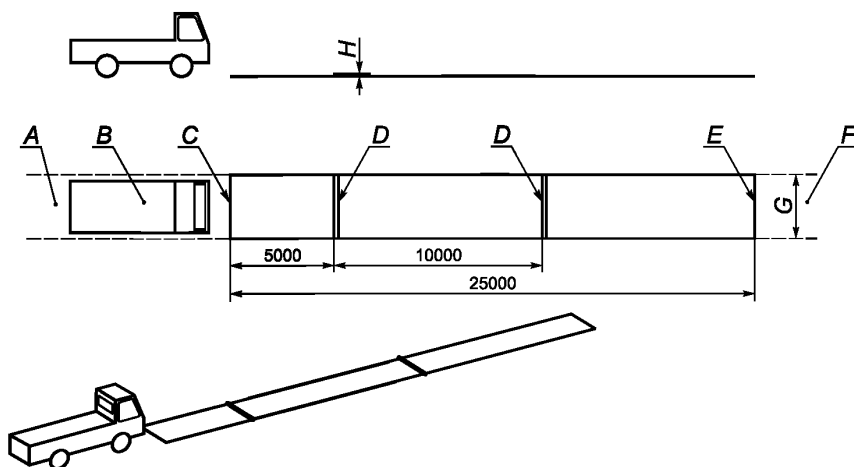
A — участок разгона; B — испытываемая машина; C — линия начала испытательного пути; D — препятствие; E — линия окончания испытательного пути; F — участок торможения; G — ширина испытательного участка; H — высота препятствия
