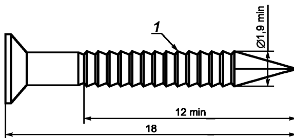
1 — не менее 13 полностью сформированных упорных кромок
