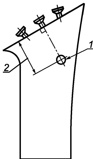
1 — просверленное технологическое отверстие под стержень диаметром 2 мм; 2 — расстояние от верхней части каблука до технологического отверстия от 20 до 25 мм
