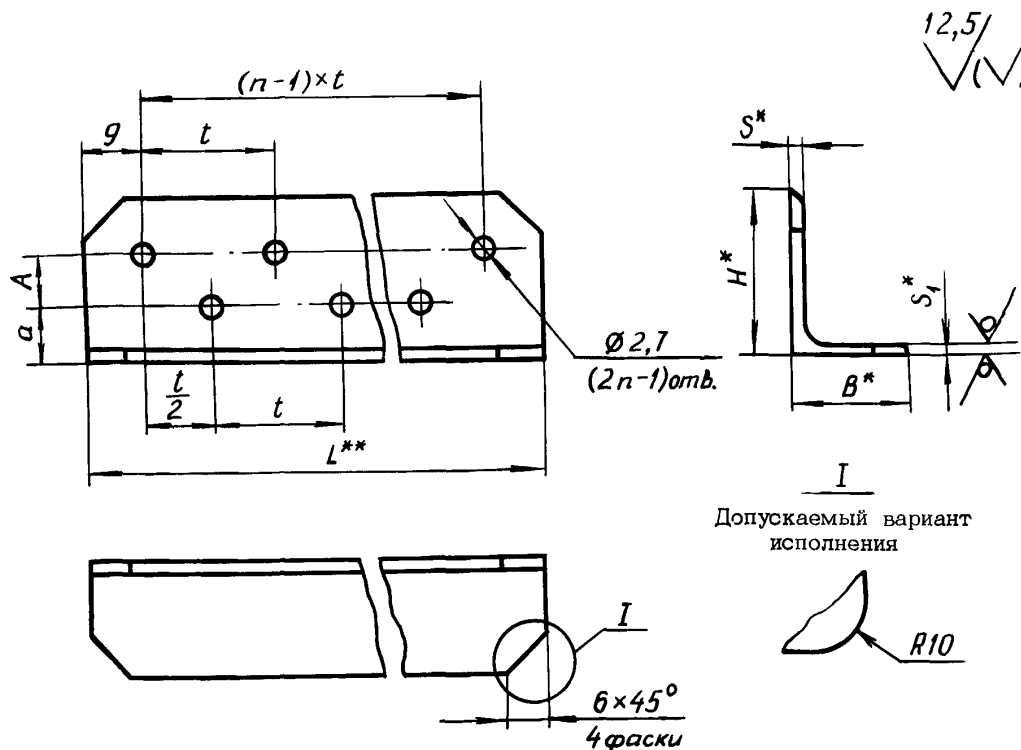
Размеры, мм
