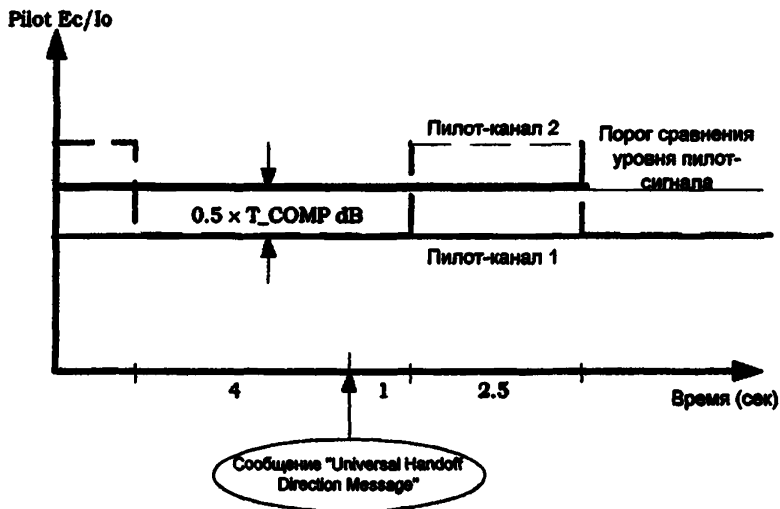
Рисунок 4.1.1-9. Уровни сигналов для проверки обнаружения пилот-канала из списка вероятных пилот-кодов (Тест 1)
