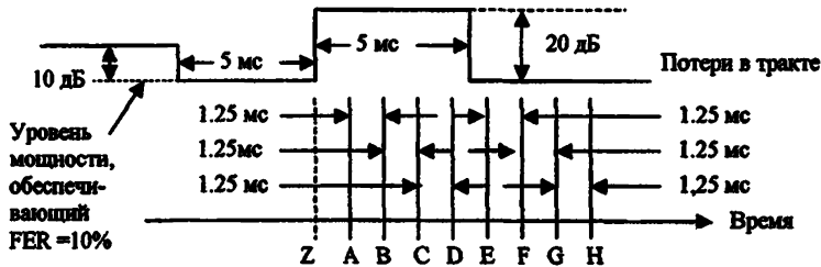
Рисунок 5.1.2-2 Временные позиции измерения отклика эмулятора АС на увеличение и снижение потерь в тракте передачи при выполнении альтернативной процедуры тестирования.
