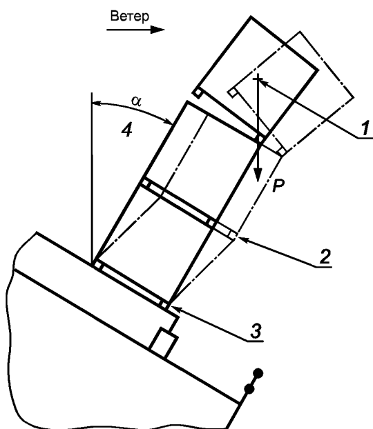
1 — опрокидывающая сила; 2 — сила перекаса; 3 — сила скольжения; 4 — качка
