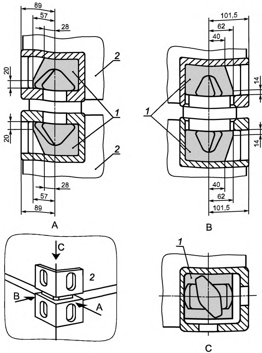
Рисунок D.7 — Ограниченная часть полости углового фитинга
