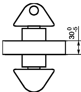
Рисунок А.6 — Промежуточная пластина
