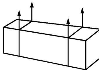
Рисунок 3 — Подъем контейнеров спредером за верхние фитинги
