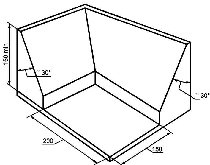
Рисунок 24 — Пример уголковой направляющей с горизонтальным упором
