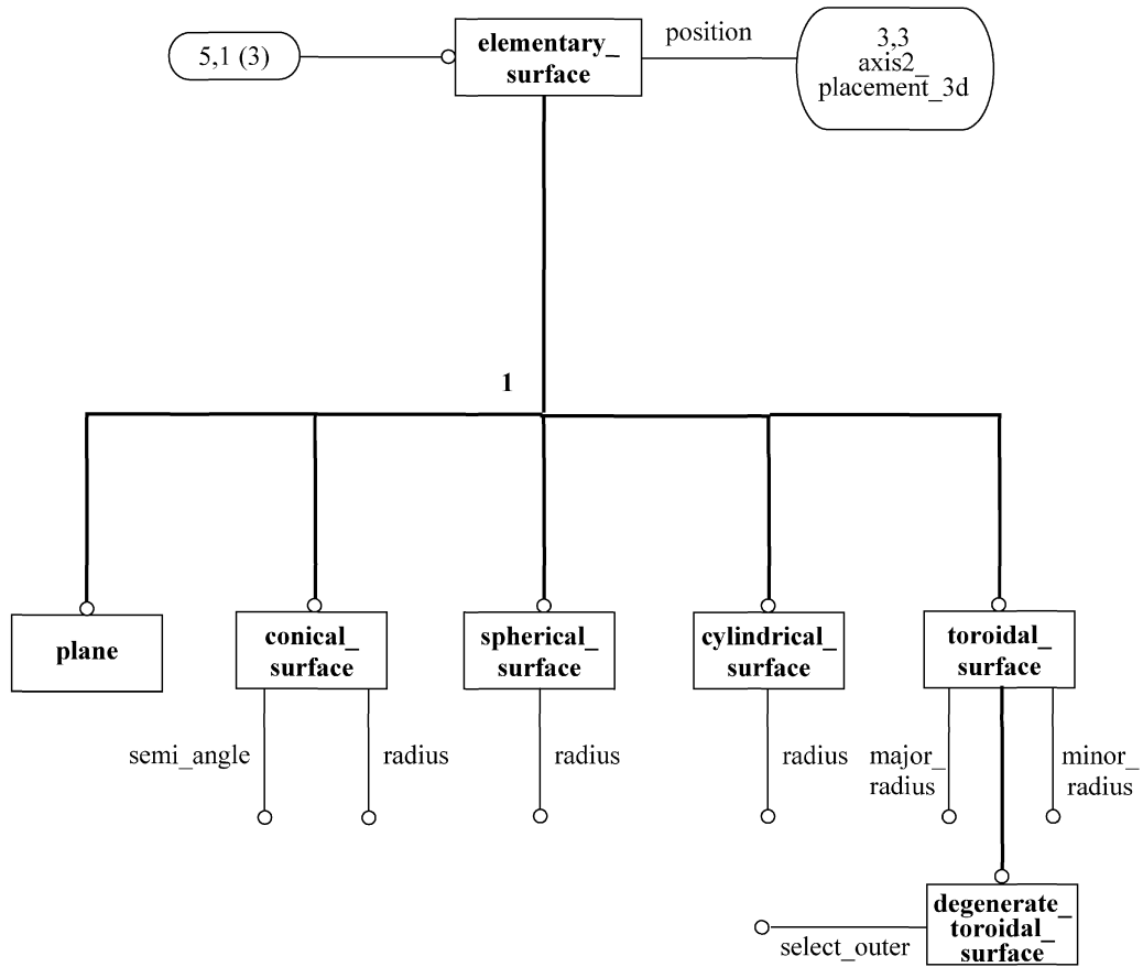
Рисунок D.5 — ПИК aic_curve_swept_solid в формате EXPRESS-G (диаграмма 5 из 9)
