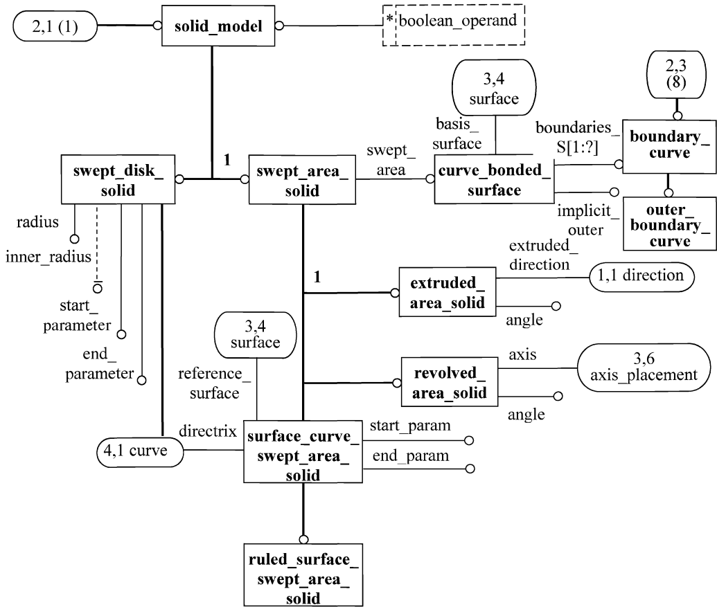
Рисунок D.2 — ПИК aic_curve_swept_solid в формате EXPRESS-G (диаграмма 2 из 9)
