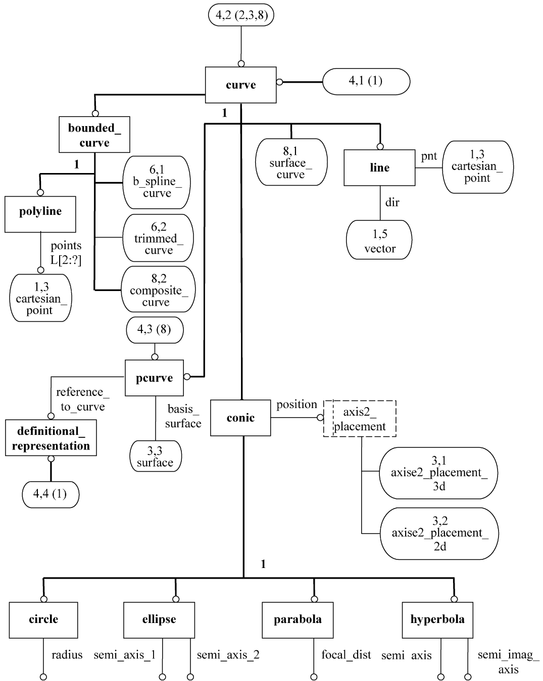
Рисунок D.4 — ПИК ic_curve_swept_solid в формате EXPRESS-G (диаграмма 4 из 9)
