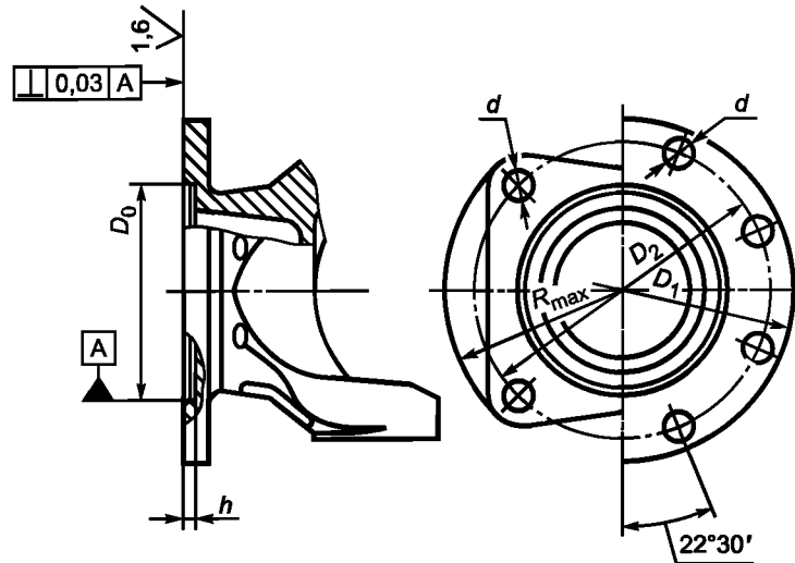
Рисунок 5 — Типы фланцев-вилок карданных шарниров с присоединительными поверхностями
