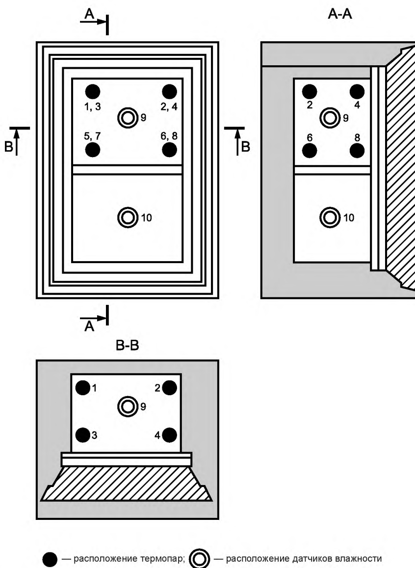
Рисунок 6 — Точки измерений (1—10) в испытуемых образцах контейнеров данных
