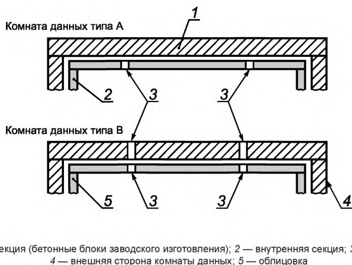
Рисунок 1 — Расположение комнаты данных при проведении испытаний (горизонтальное сечение)
