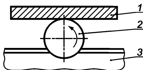
1 — образец; 2 — валик; 3 — битум
