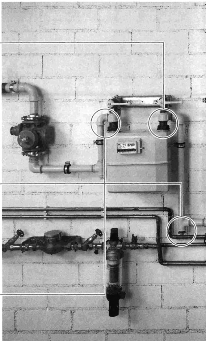
Проведение основных тестов с использованием прибора testo 312-2/3
