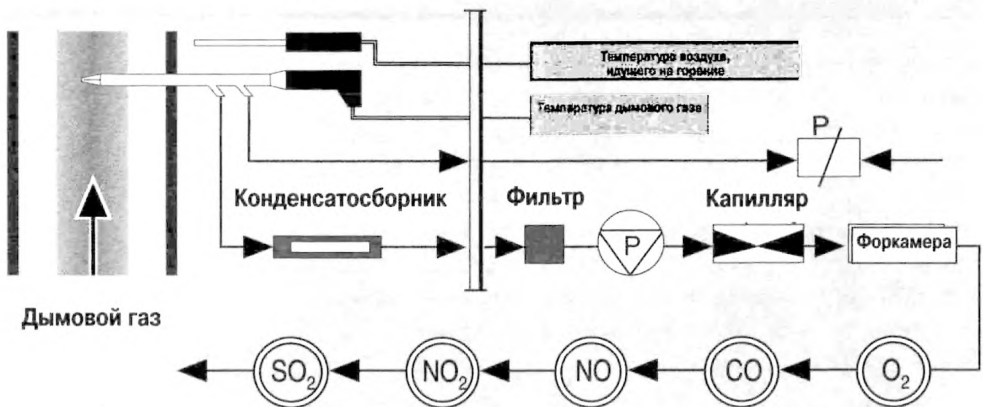
Рис. 31: Упрощённая схема газового тракта в анализаторе дымового газа
