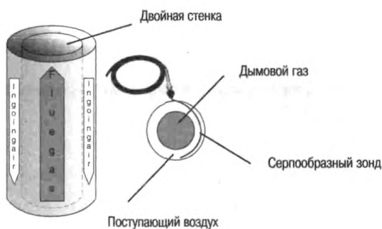
Рис. 20: Замер уровня O_2 в межстенном пространстве дымохода серпообразным зондом
