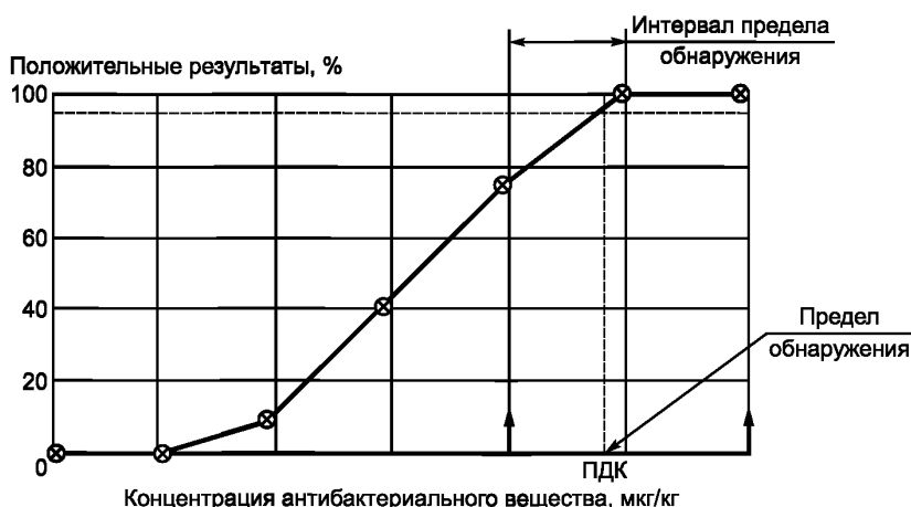
Рисунок 1 — Модель кривой содержание/сигнал для определения предела обнаружения
