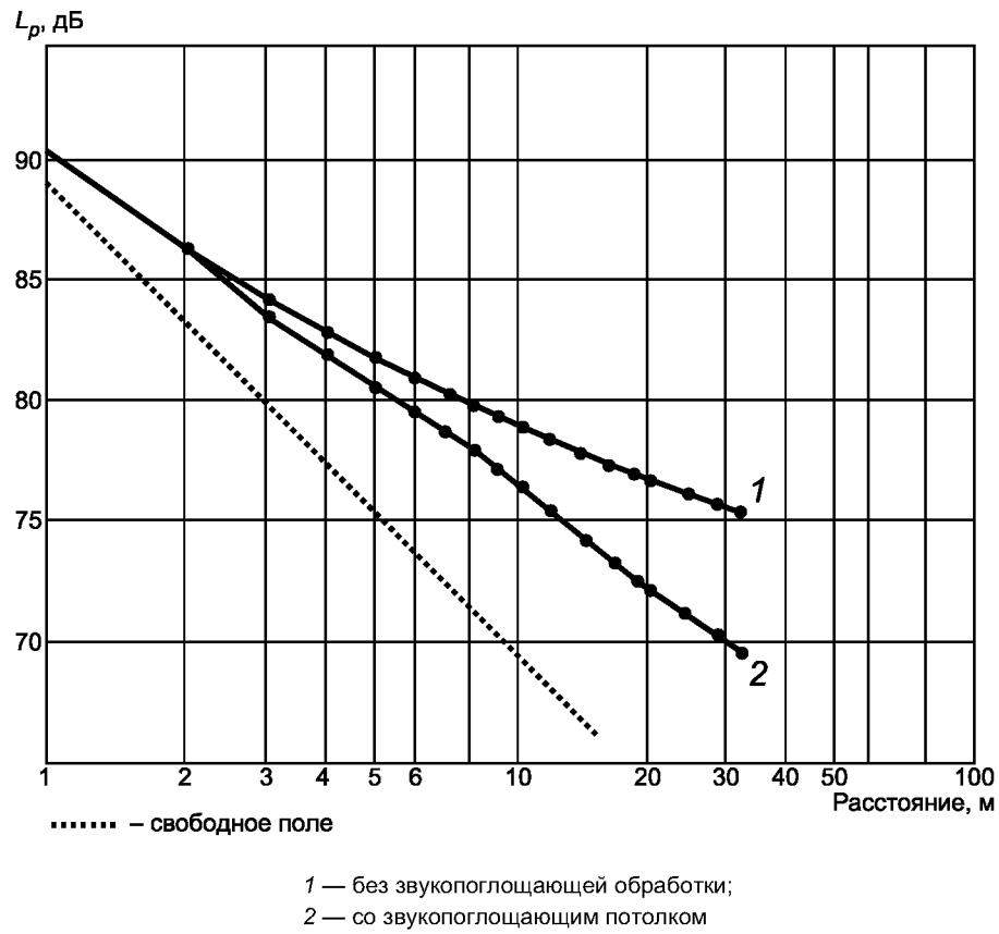
Рисунок D.1 — Рассчитанные линии пространственного распределения звука
