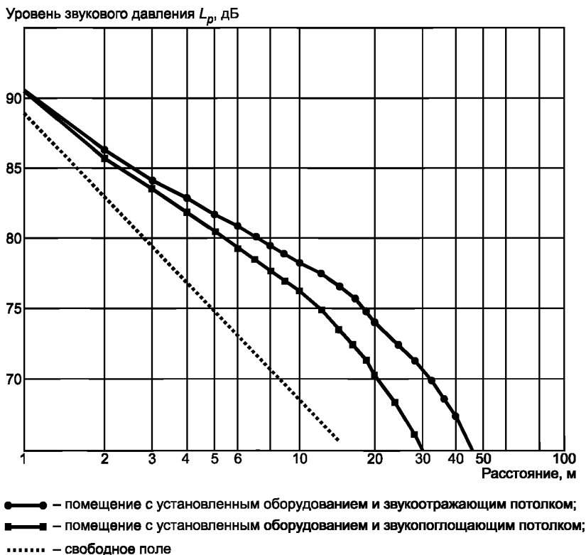
Рисунок 2 — Типичные линии пространственного распределения звука, излученного ненаправленным точечным источником звуковой мощностью 100 дБ в плоском заполненном оборудовании помещения со звукопоглощающим и со звукоотражающим потолком
