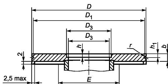
Рисунок 2 — Опорный фланец
