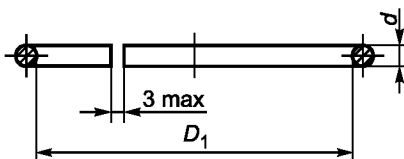
Рисунок 4 — Установочное кольцо
