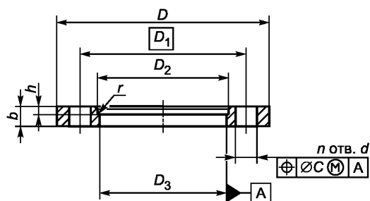
Рисунок 3 — Накладной фланец
