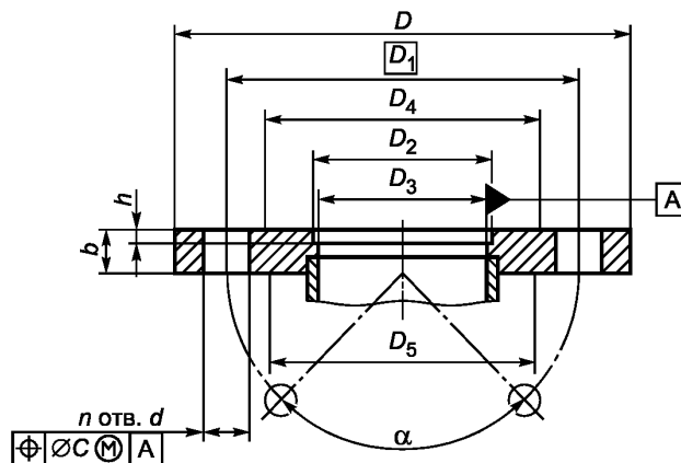
Рисунок 1 — Неподвижный фланец
