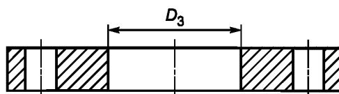
Рисунок Б.1 — Расточка фланца
