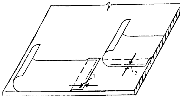
Рисунок 5 — Допускаемые отклонения при устройстве двухслойной рулонной кровли:
