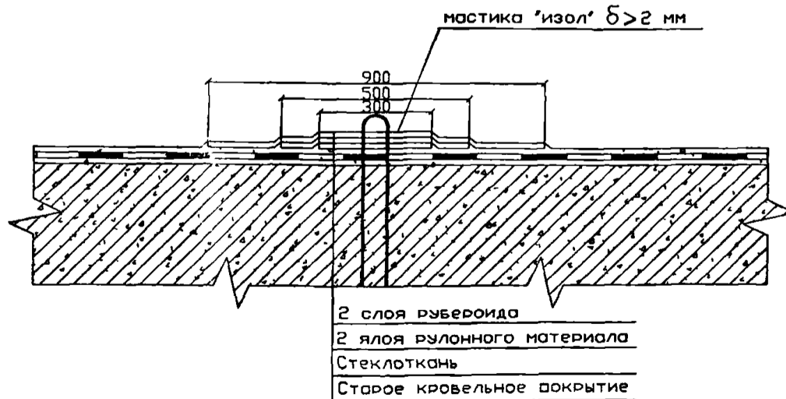
Рисунок 2 (продолжение) — Устройство мест примыкания
