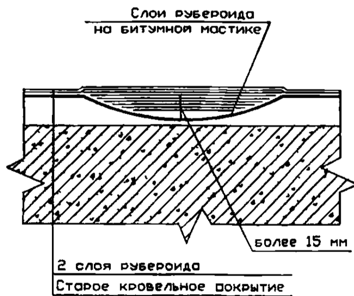
Рисунок 1 — Ремонт кровельного ковра
