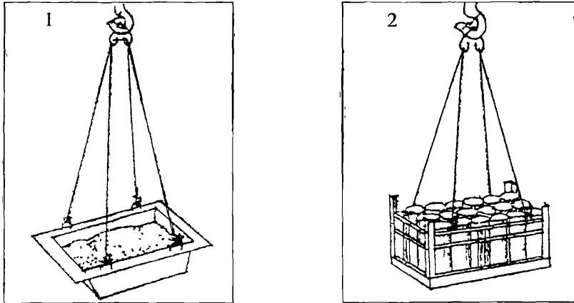
Рисунок 6 — Схемы строповок
