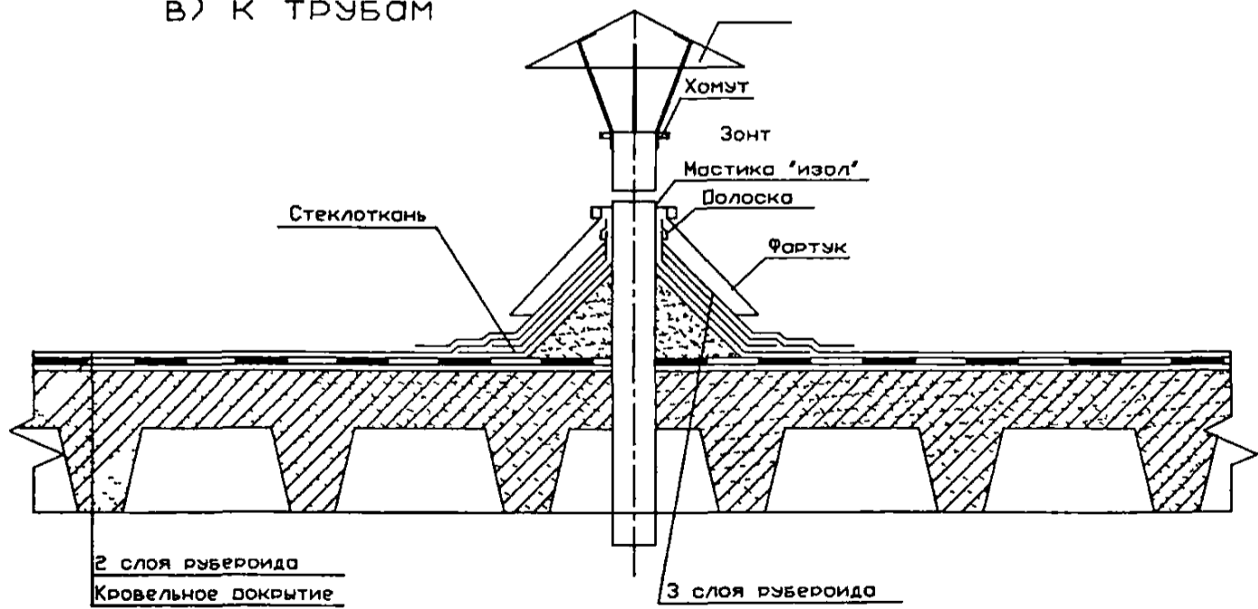
Рисунок 2 — Устройство мест примыкания
