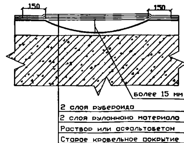
Рисунок 1 — Ремонт кровельного ковра
