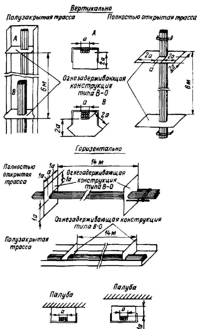
Рис. 16.8.4.3.2-2 Защита кабельных трасс огнезадерживающими конструкциями типа В-О
