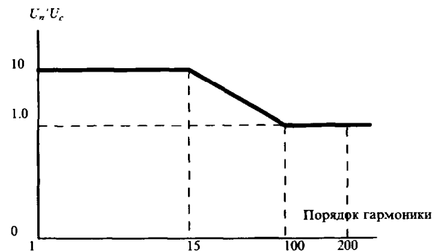
Рис. 2.2.1.2.2 График высших гармоник сети
