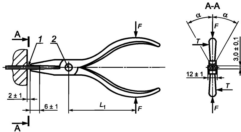
1 — образец для испытания; 2 — ось шарнира
