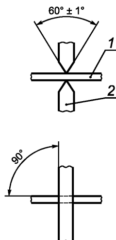
1 — калибруемая проволока; 2 — твердосплавный резец
