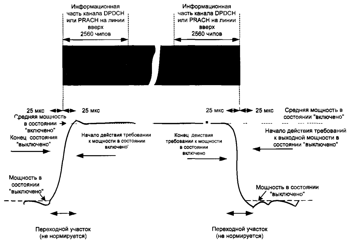
Рисунок 1. Шаблон включения и выключения излучения передатчика во времени для физического канала произвольного доступа
