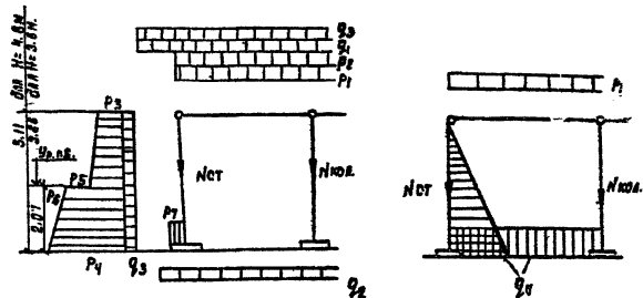
Рис.1 Схемы основных сочетаний нагрузок.
