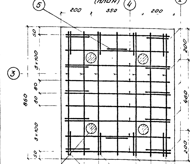
Вид В (план)
