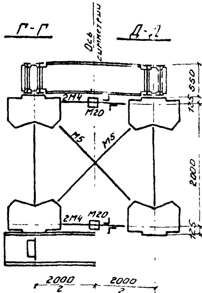
Спецификация УЦКМ-60 (для моста отв. 5,0м)
