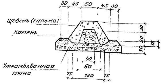
Б-Б
