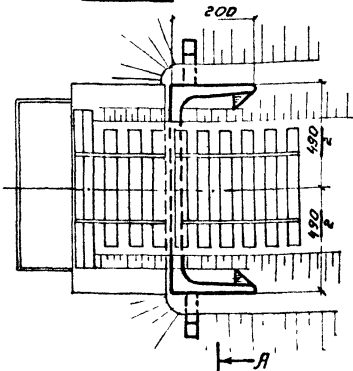
План
