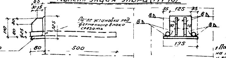
Конструкция упора (М10)
