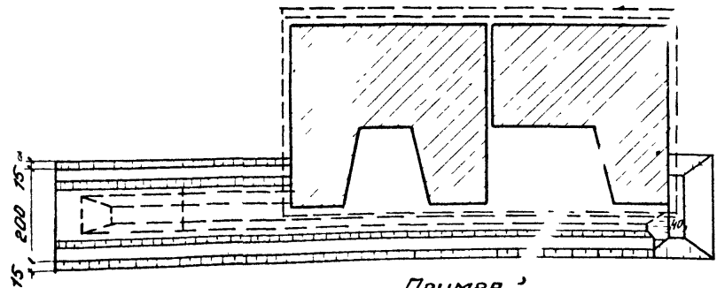
ПРИМЕР 2 Разрез по оси пути
