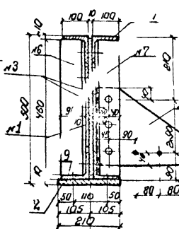
С-И
