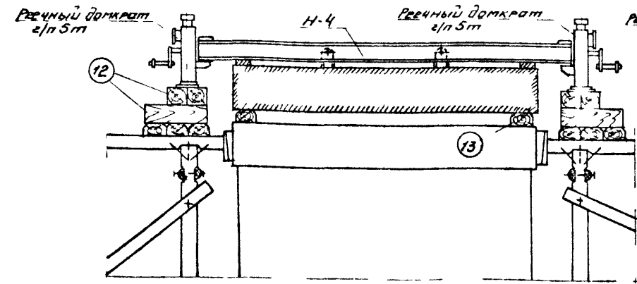
Схема моста
