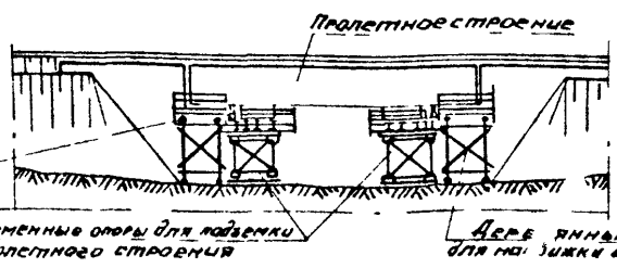
Схема моста
