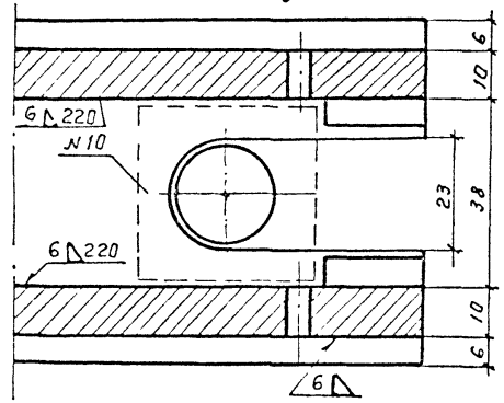
Вид А (Вид снизу)
