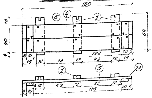
Бортовой щит
