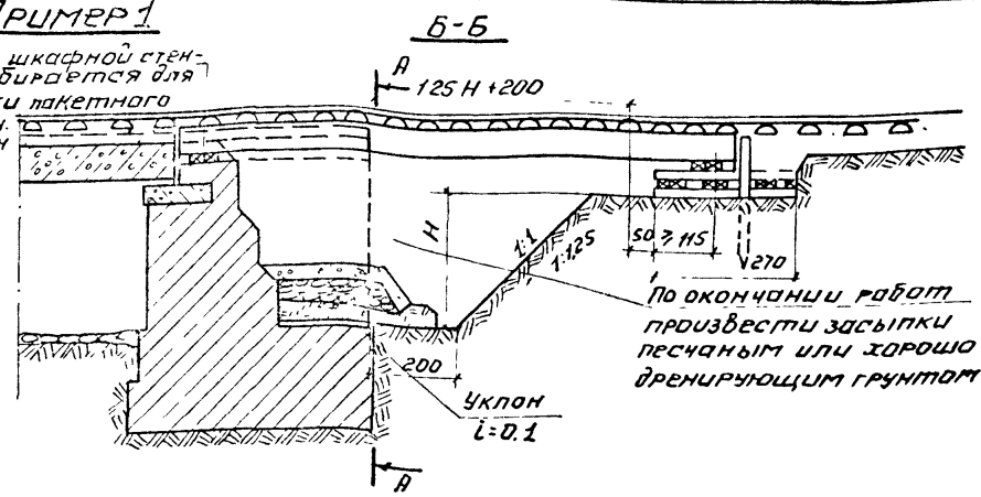
Б-Б
