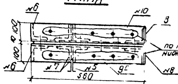
А-А
