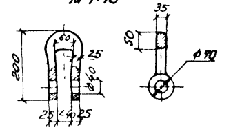
Прикрепление такелажной скобы к балкам раостверка
