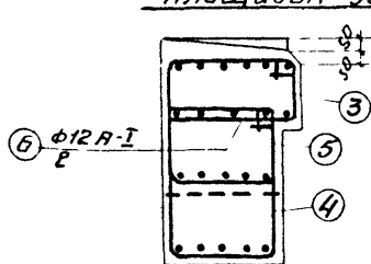
Нарощивание шкафной стенки и прикрепление надстенного бруса
