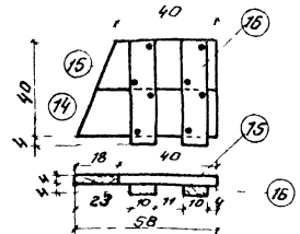
Щитовой щит
