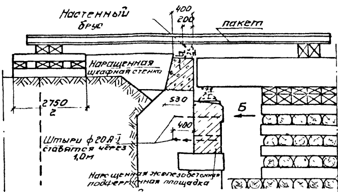
Армирование подферменных площадок устоев
