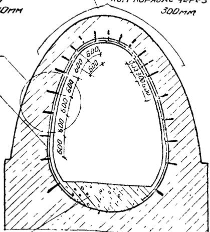
Повышение лотка бетонной кладкой М200
