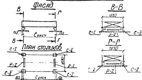
Монтажная схема
