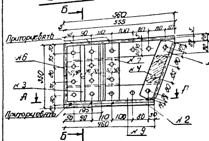
ПЛАН
