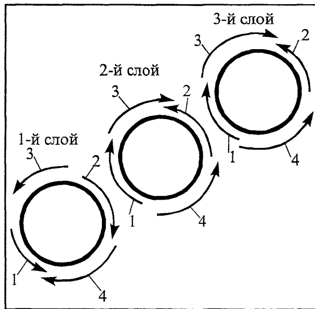
Рисунок 2 – Порядок наложения слоев шва при сварке стыка
