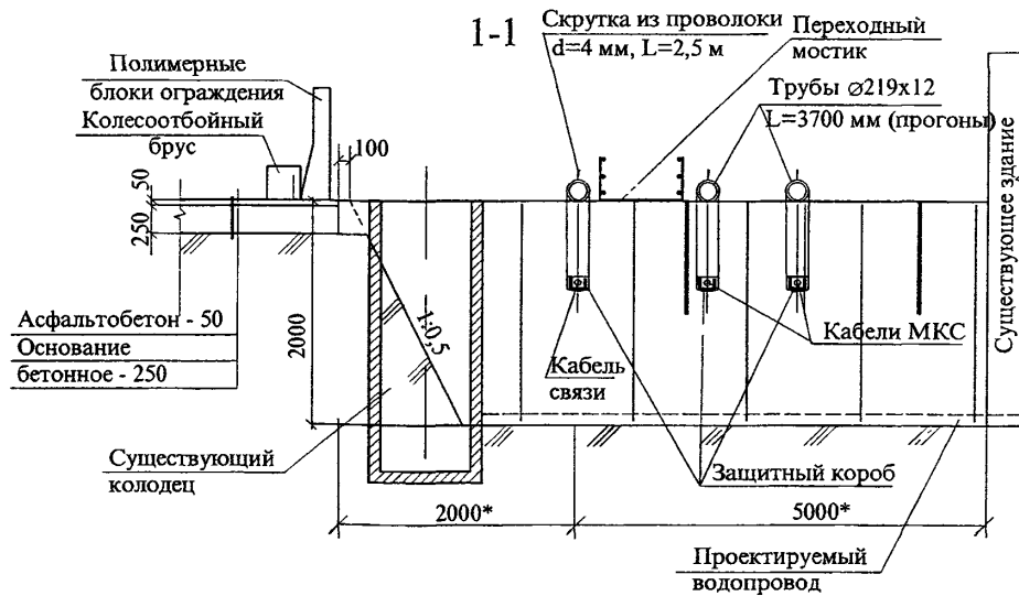
Рисунок 6 – Примерная схема пересечения трубопровода с кабелями связи и МКС
