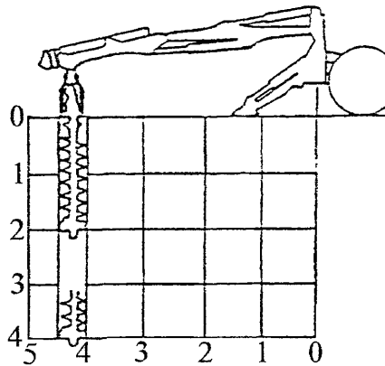
Рисунок 2– Схема бурения скважины под опору
