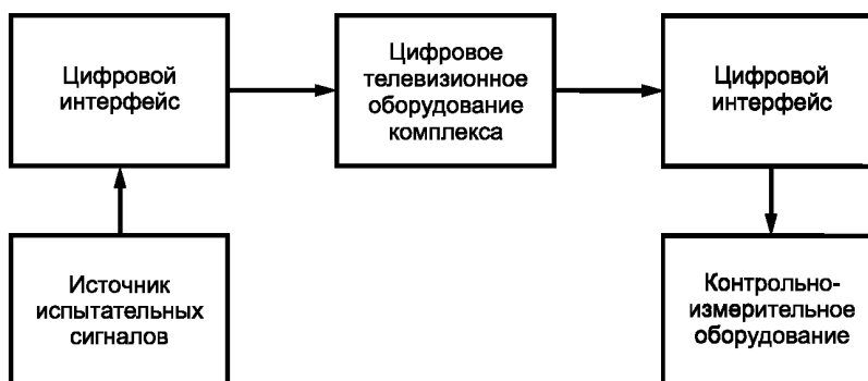
Рисунок 3 — Схема измерения параметров студийного (внестудийного) комплекса
