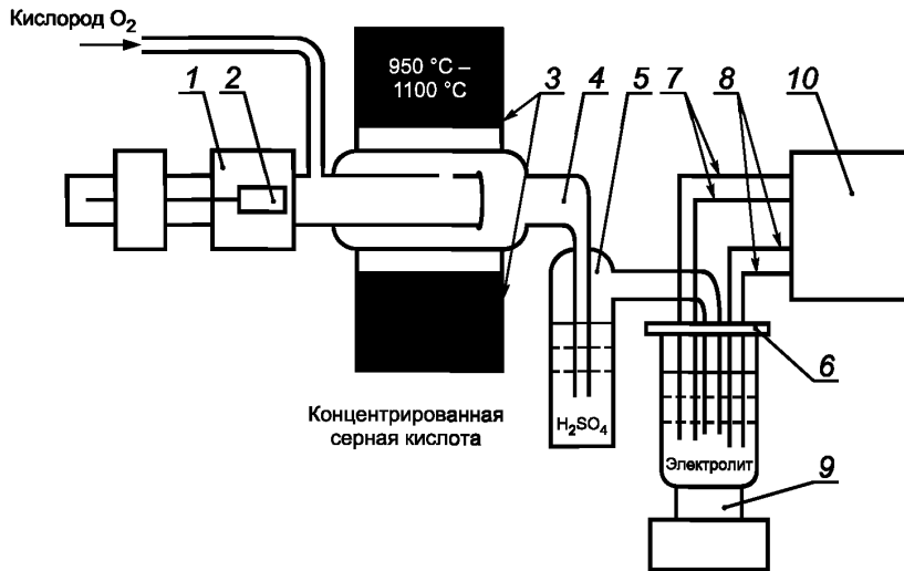
1 — приемник образца; 2 — кварцевая лодочка; 3 — печь для сжигания; 4 — кварцевая трубка для сжигания; 5 — абсорбер с концентрированной серной кислотой; 6 — ячейка с электролитом; 7 — рабочие электроды; 8 — измерительные электроды; 9 — электромагнитная мешалка; 10 — регистрирующее устройство для регистрации массы ионов хлора
