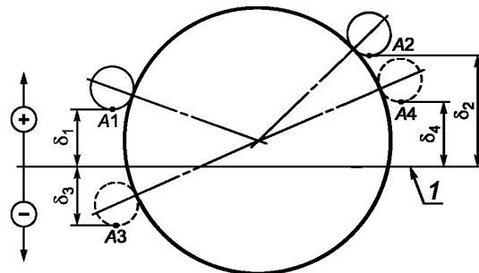
1 — линия номинального положения контрольных точек замков, наносимая на шаблон; \delta — измеряемое по вертикали отклонение замка от номинального положения; А1, А2 — контрольные точки первого торца; А3, А4 — контрольные точки второго торца; А1, А3 — контрольные точки первого замка; А2, А4 — контрольные точки второго замка
