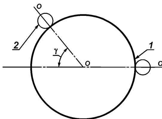
O — O — ось шпунтовой стены; \gamma — угол поворота оси ряда
