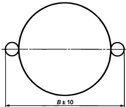
Рисунок 4 — Предельное отклонение ширины шпунтового профиля
