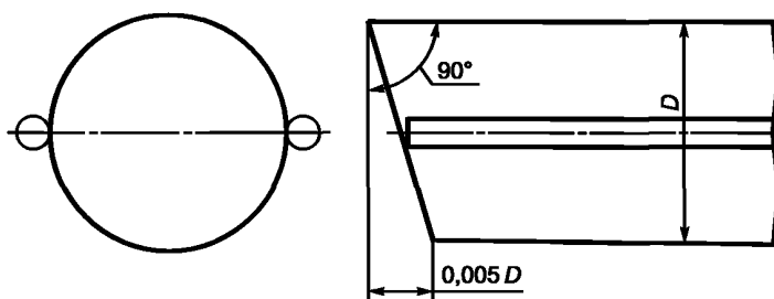
Рисунок 6 — Предельный перекос плоскости торца шпунтового профиля
