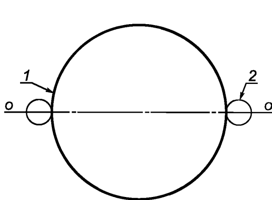
1 — труба; 2 — замок; O — O — ось шпунтовой стены
