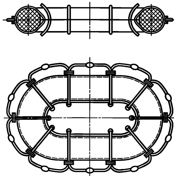
Рисунок 1 — Спасательный прибор
