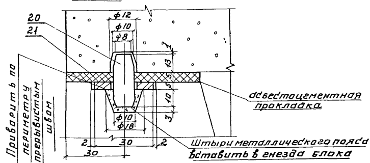
Узел "А"
