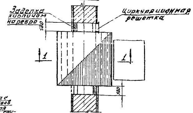
План
