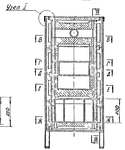
РАЗРЕЗ I-I
