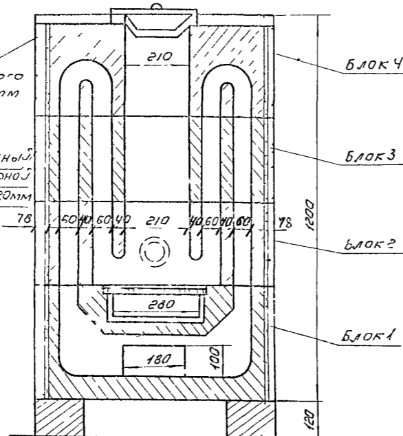
РАЗРЕЗ II-II
