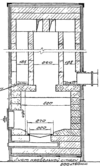
Разрез I-I
