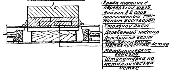
Разрез 2-2
