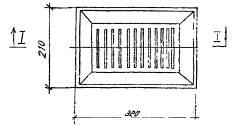
План
