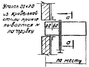
Дымоход патрубок с задвижкой вид сверху
