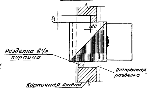
План IV-IV
