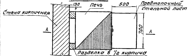
План II-II
