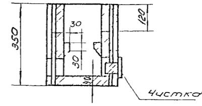
РАЗРЕЗ Б-Б
