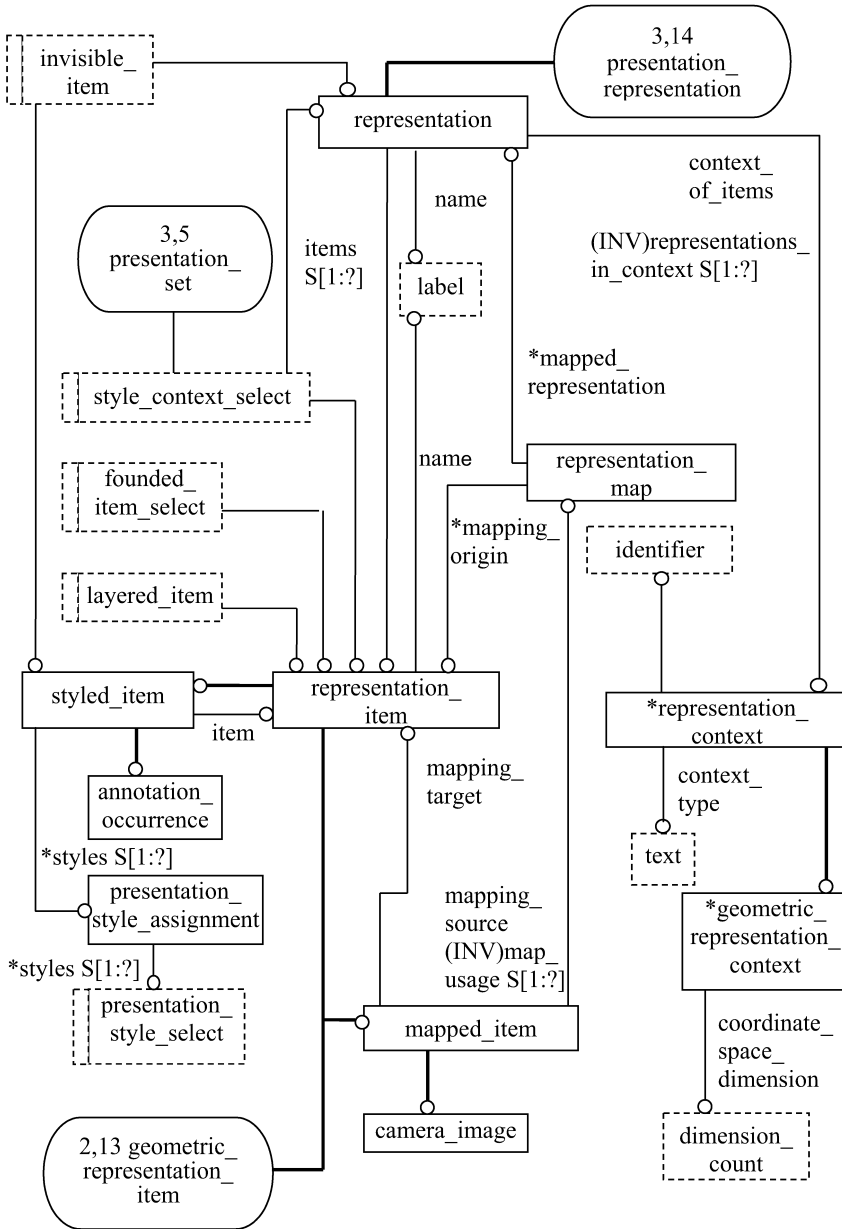
Рисунок С.1 — Расширенный листинг ПИК — EXPRESS-G диаграмма 1 из 14
