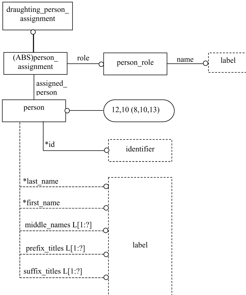
Рисунок С.12 — Расширенный листинг ПИК — EXPRESS-G диаграмма 12 из 14
