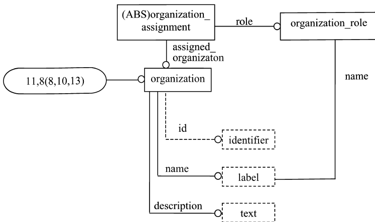
Рисунок С.11 — Расширенный листинг ПИК — EXPRESS-G диаграмма 11 из 14
