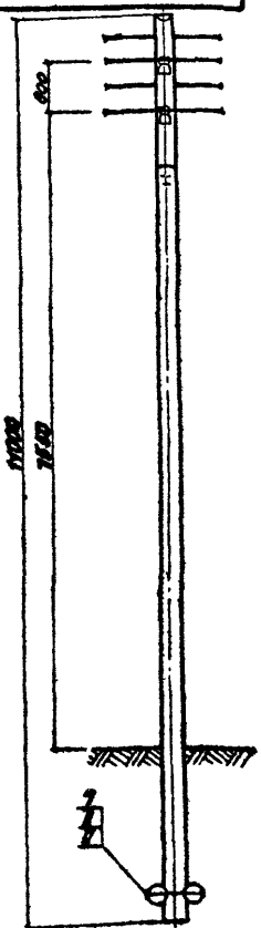
Схема крепления проводов на ут. пром. промежуточной опоре
