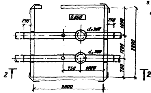
Камера выпуска воздуха План
