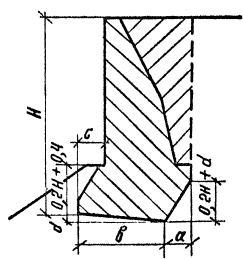
Расчетная схема.
