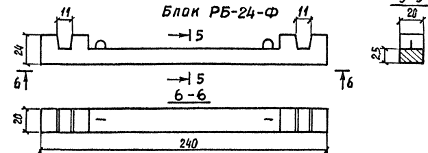
Блоки РБ-20...55
