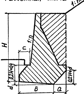
Расчетная схема
