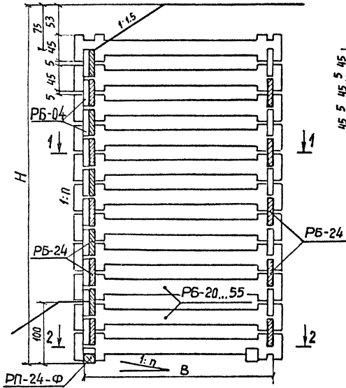
Общий вид стены (М 1:50) Поперечный разрез
