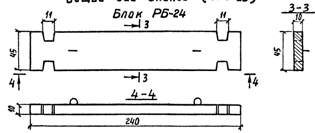
Блок РБ-24-Ф
