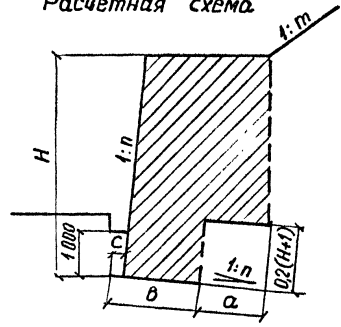
Расчетная схема
