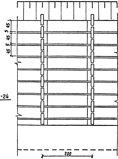
Общий вид стены (М 1:50) Поперечный разрез
