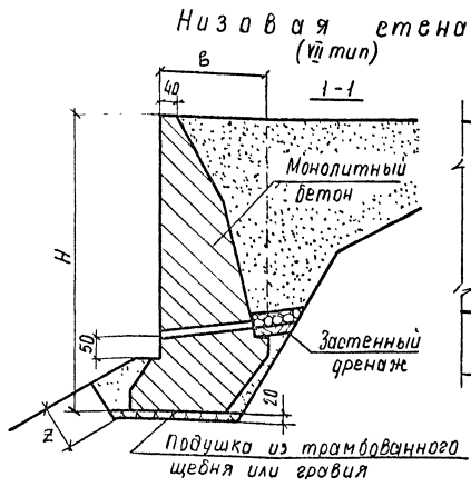
Устройство застенного дренажа
