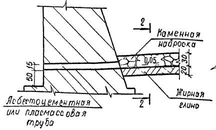
Устройство застенного дренажа
