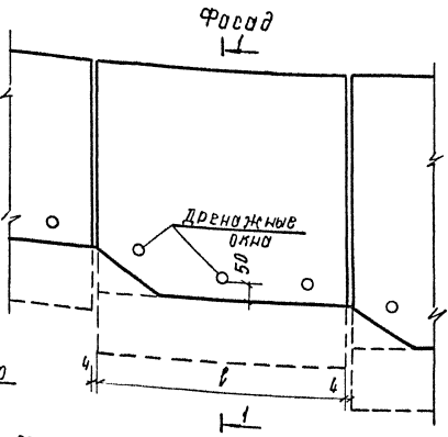
Устройство застенного дренажа
