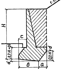
Расчетная схема
