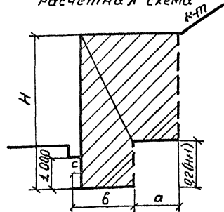
Расчетная схема
