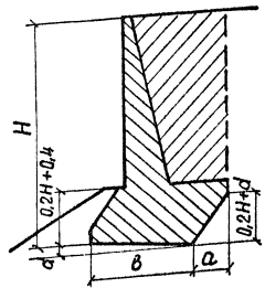
Расчетная схема
