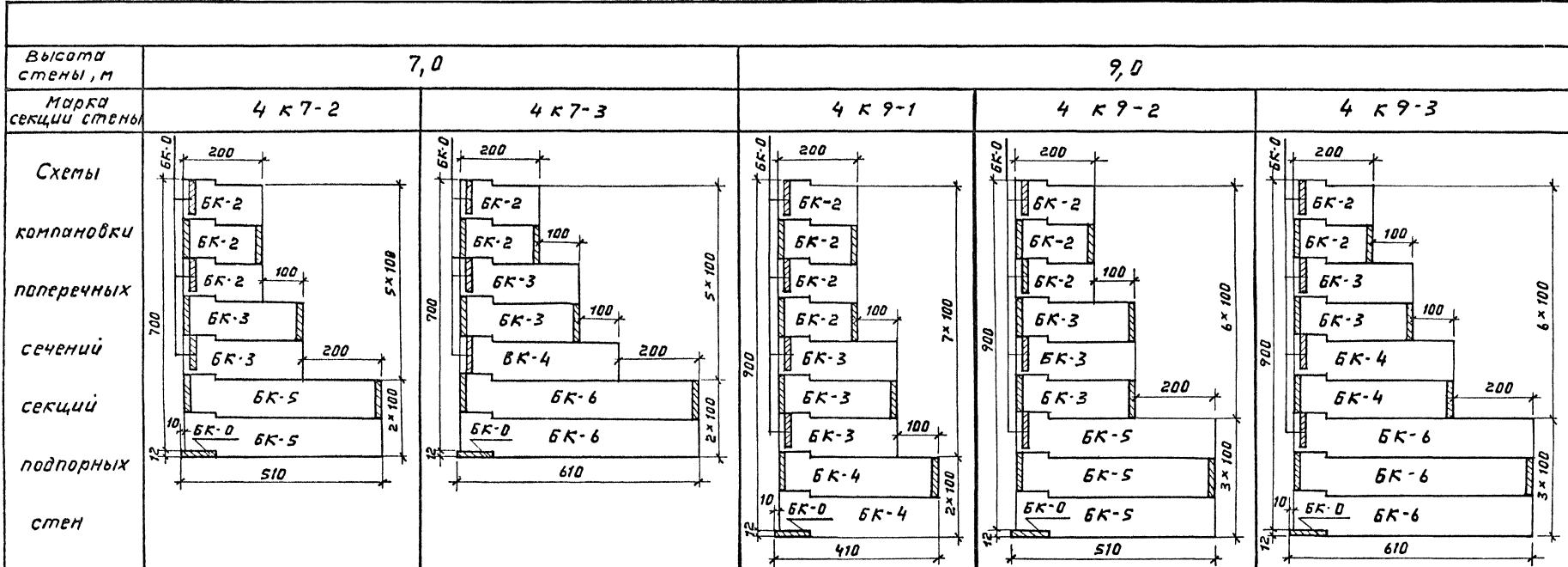
Расход монтажных элементов и материалов на секцию (10 п. м.) подпорной стены
