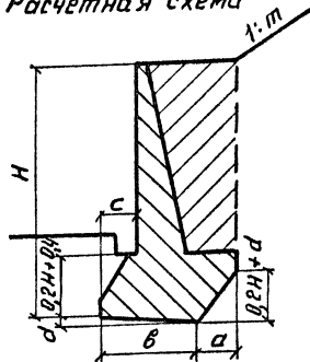
Расчетная схема
