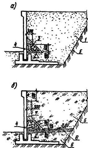
Рис. 2. Схема дренажа
