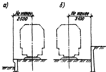
Рис.1. Габариты приближения железнодорожного пути нормальной колеи при расположении: а) - с верхней стороны стены; б) - с нижней.
