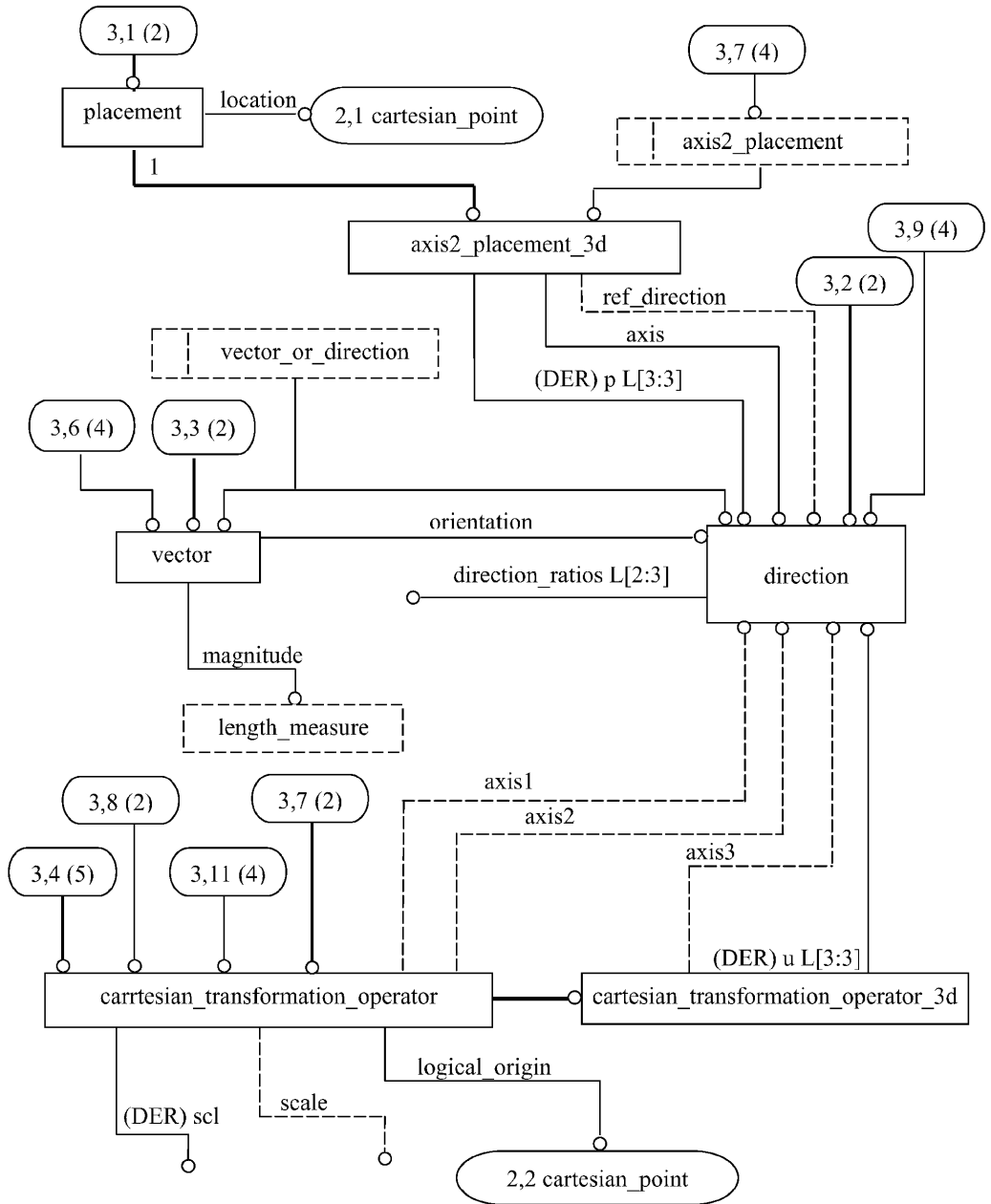
Рисунок С.3 — aic_shell_based_wireframe — EXPRESS-G диаграмма 3 из 6
