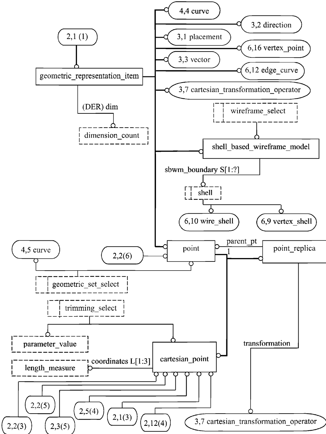
Рисунок С.2 — aic_shell_based_wireframe — EXPRESS-G диаграмма 2 из 6
