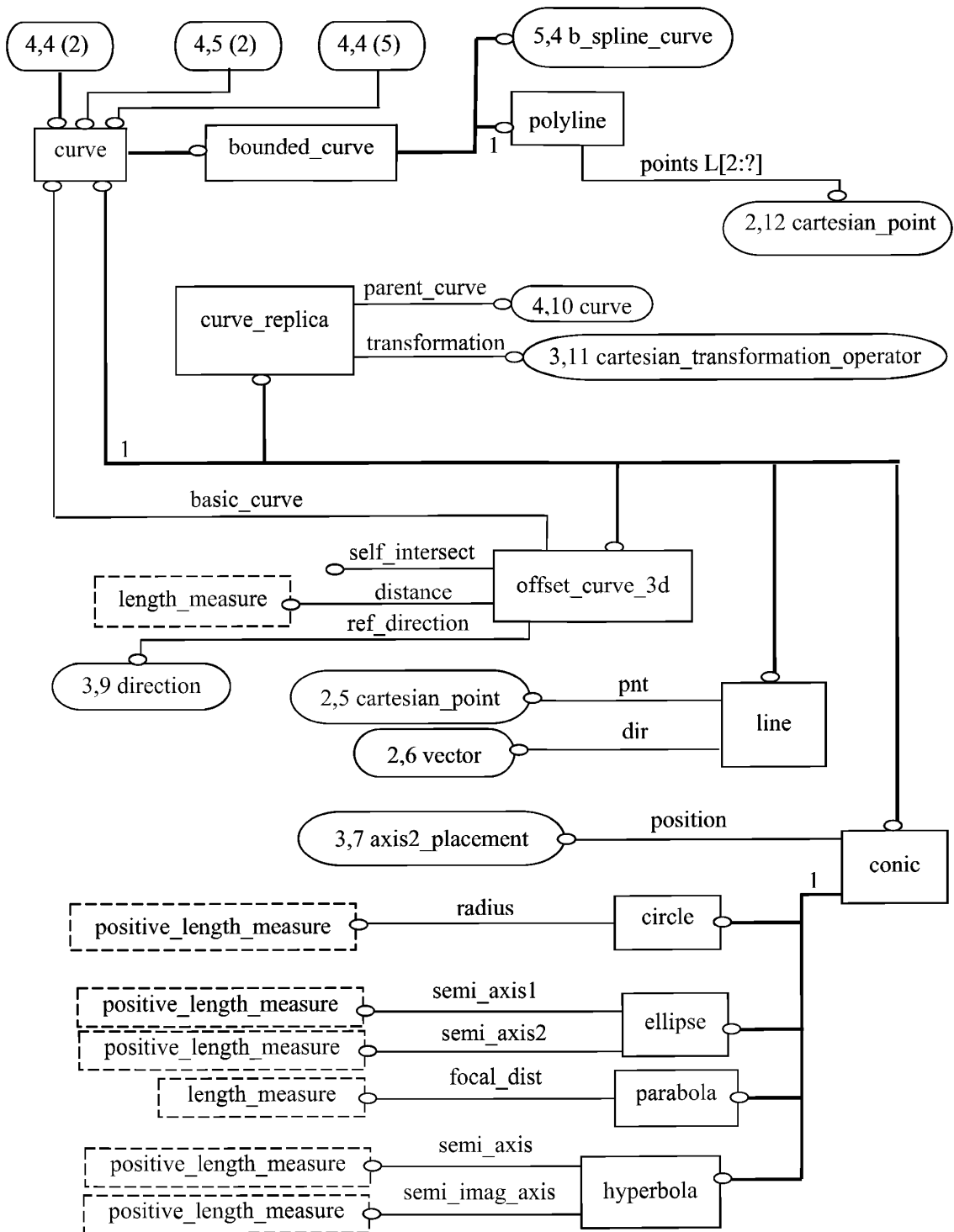
Рисунок С.4 — aic_shell_based_wireframe — EXPRESS-G диаграмма 4 из 6
