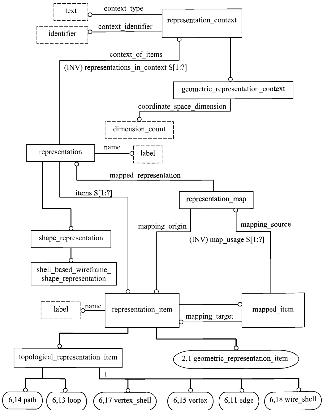
Рисунок С.1 — aic_shell_based_wireframe — EXPRESS-G диаграмма 1 из 6
