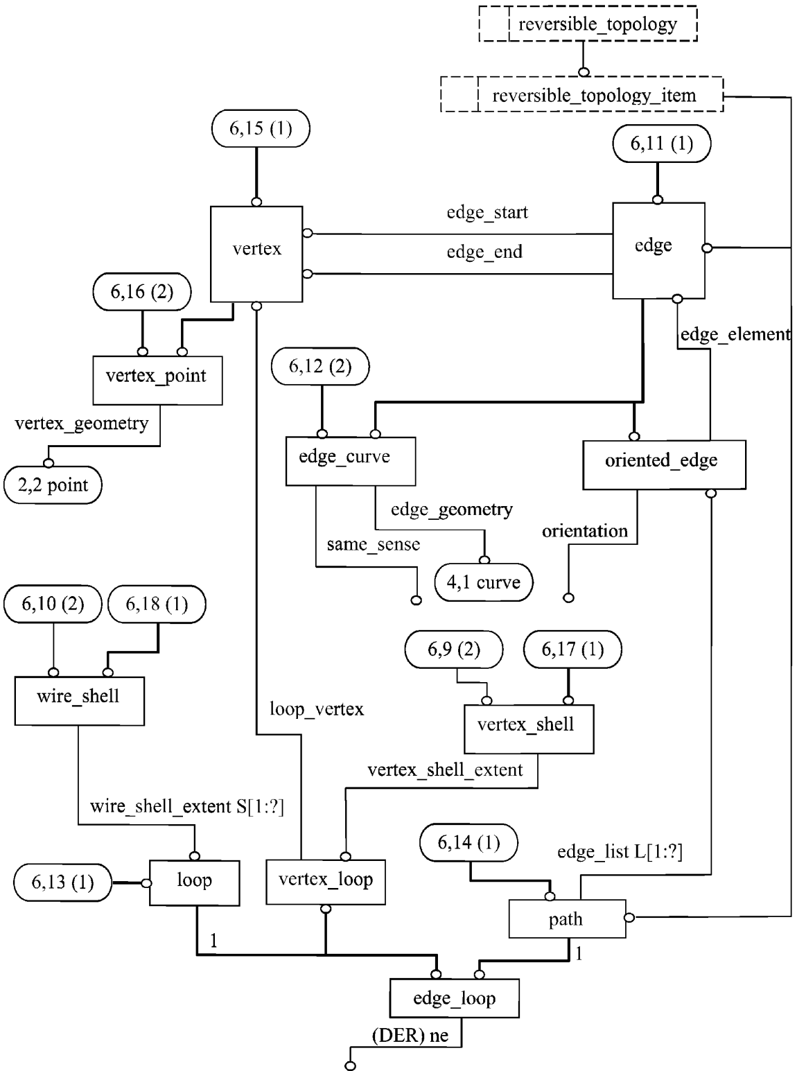
Рисунок С.6 — aic_shell_based_wireframe — EXPRESS-G диаграмма 6 из 6
