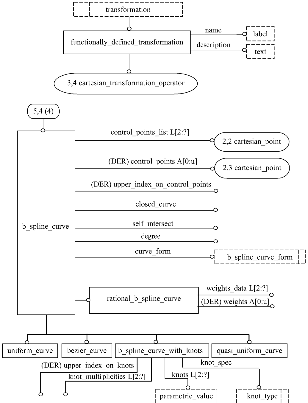
Рисунок С.5 — aic_shell_based_wireframe — EXPRESS-G диаграмма 5 из 6
