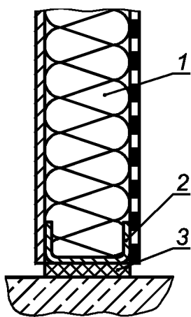
а) Резиновая опора
