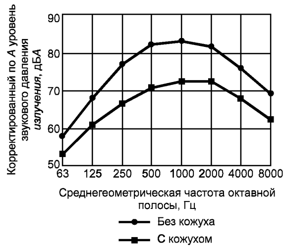
Рисунок В.7 — Спектр скорректированных по А уровень звукового давления излучения на рабочем месте оператора гофрировочной машины
