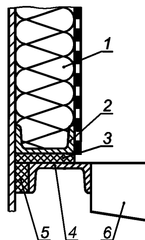
с) Резиновая опора на поддерживающем профиле
