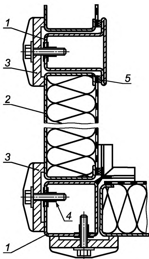
1 — каркас; 2 — стенка; 3 — зажим; 4 — закладная гайка; 5 — резиновое уплотнение
