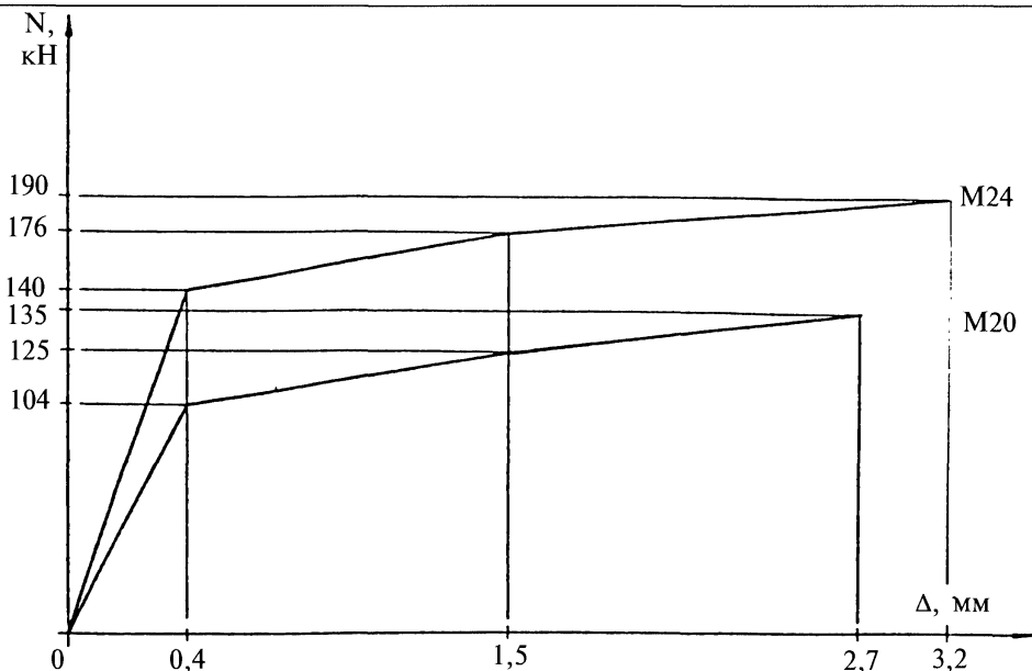
Рис. 2.5. Зависимости между усилиями сдвига и перемещениями сдвига и изгиба стержней болтов класса прочности 8,8
