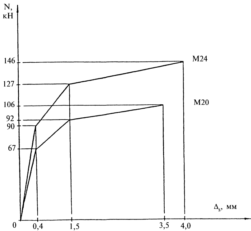
Рис. 2.4. Зависимости между усилиями сдвига и перемещениями сдвига и изгиба стержней болтов класса прочности 5.8
