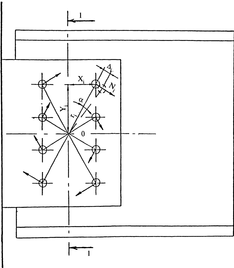
Рис. 2.2. Схема распределения усилий между болтами в срезном соединении
