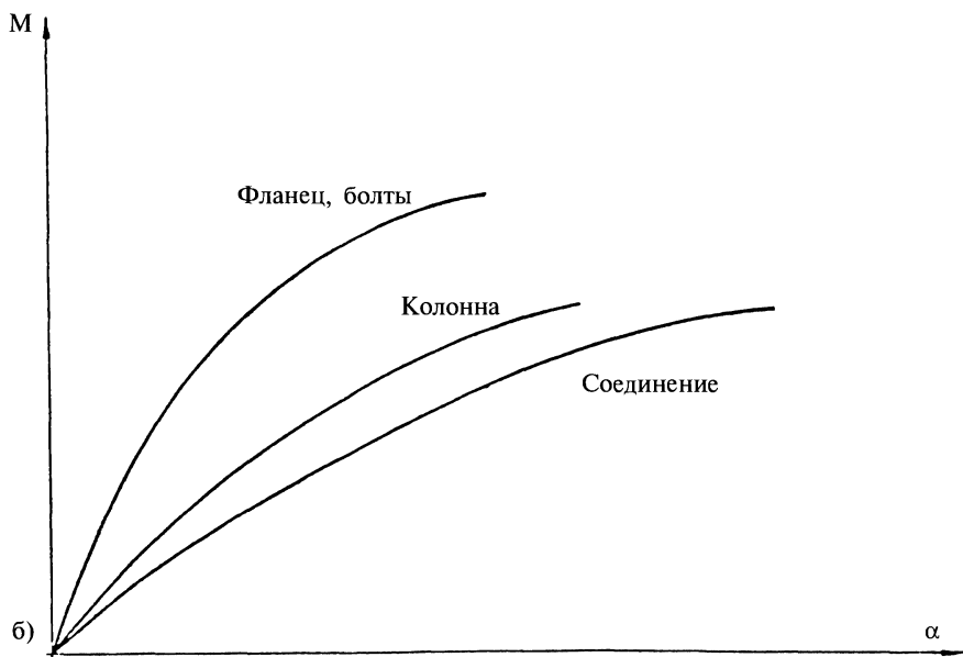
Рис. 1.2. Вклад опорной части колонны в деформативность изгибаемого фланцевого соединения
