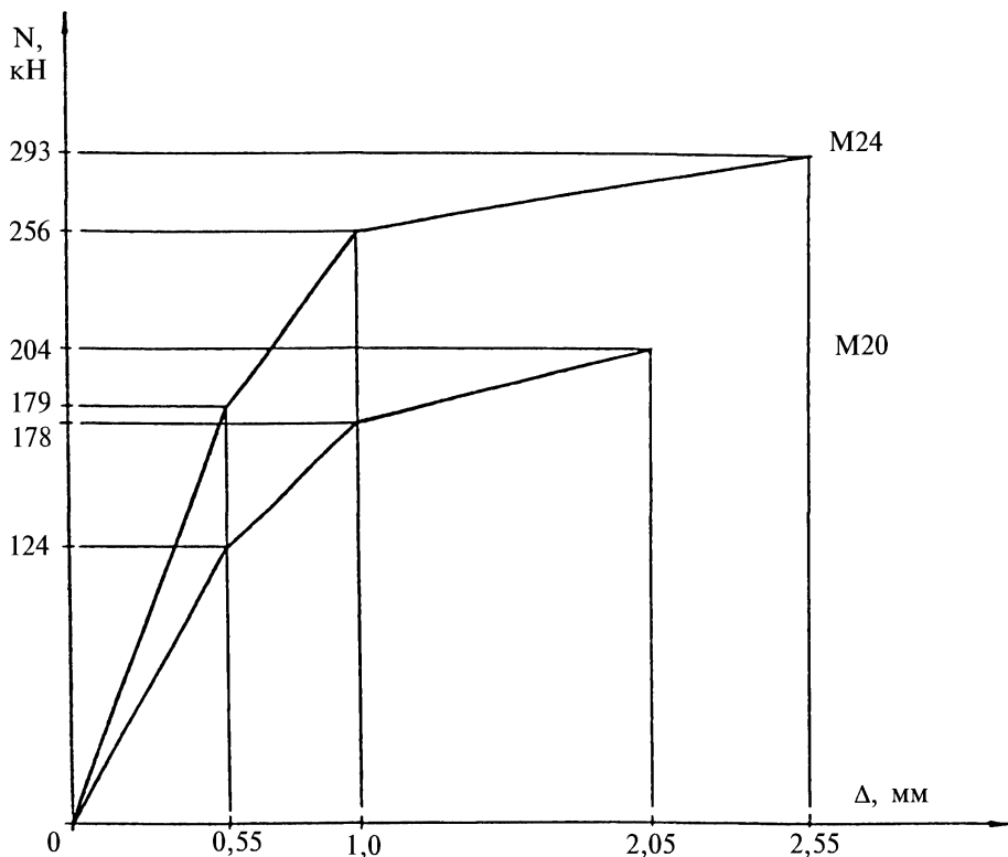
Рис. 2.6. Зависимости между усилиями сдвига и перемещениями сдвига и изгиба стержней высокопрочных болтов
