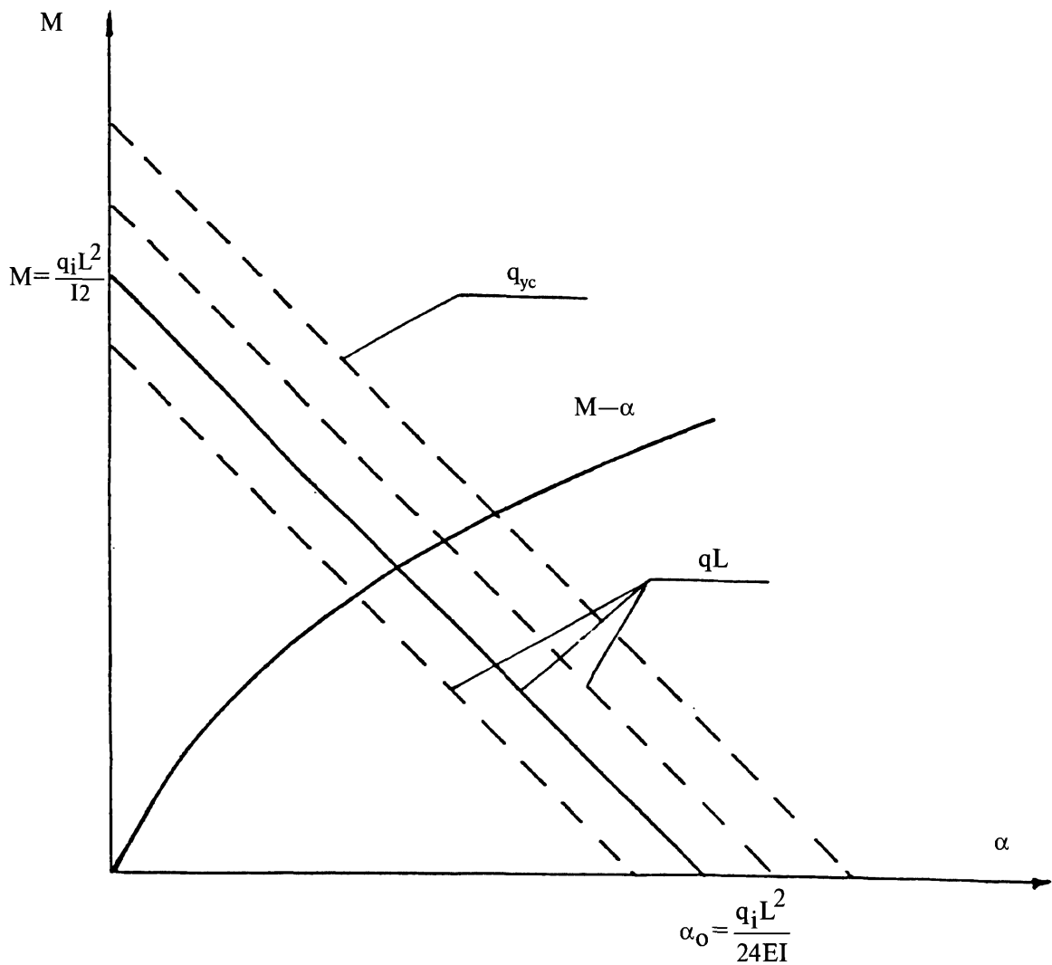
Рис. 1.3. Кривая «М— \alpha » соединения и балочная линия для постоянной нагрузки
