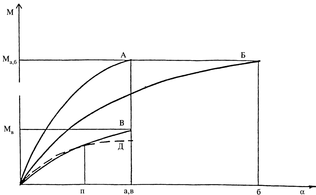
Рис. 1.1. Диаграммы «момент — угол поворота» соединений различной конструктивной формы
