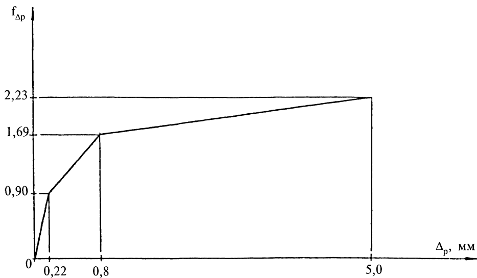
Рис. 2.3. Зависимость коэффициента f_{\Delta p} от перемещений смятия \Delta_p
