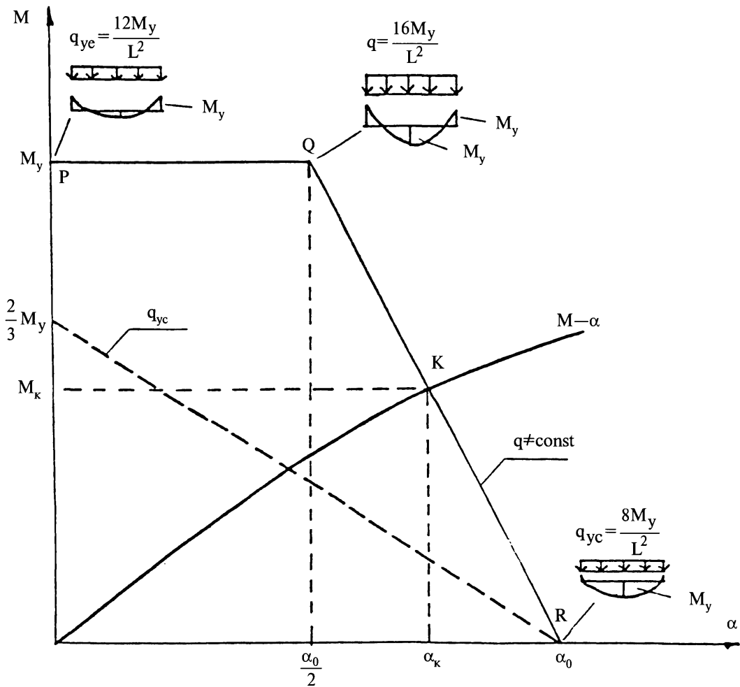
Рис. 1.4. Кривая «М-α» соединения и балочная линия PQR, соответствующая постоянному уровню напряжений текучести
