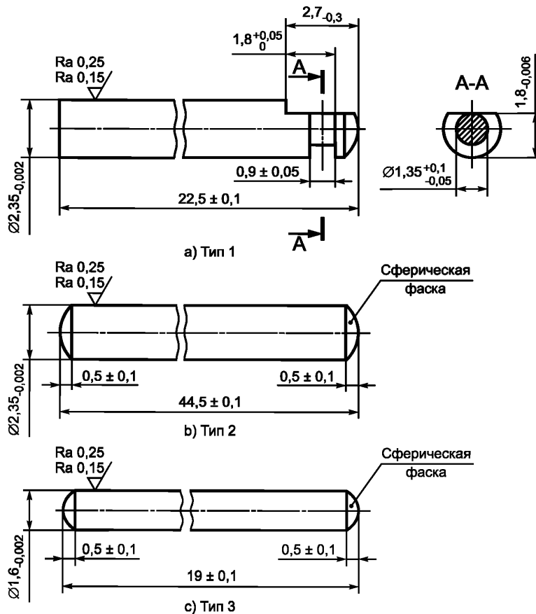
Рисунок 2 — Контрольные оправки
