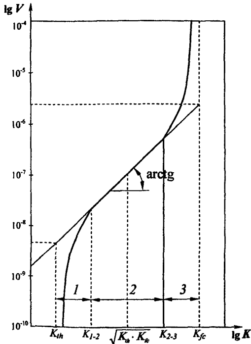
Рис. П.10.1. Типичная кинетическая диаграмма усталостного разрушения. 1, 2, 3 - участки диаграммы.
