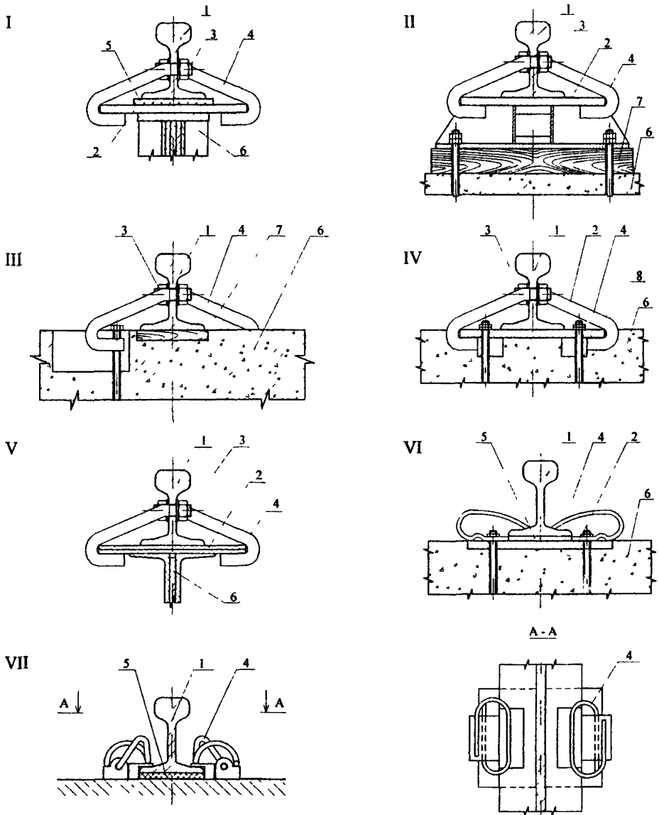
Рис. П.5.8. Промежуточные крепления для направляющей, установленной на стальной (I, V, VII) и железобетонной (II, III, IV, VI) балке craneвого пути.
