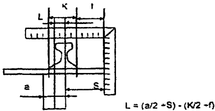
Рис. П.8.3. Определение расстояния от грани рельса до верхнего пояса балки кранового пути. Стальной угольник устанавливается по уровню.
