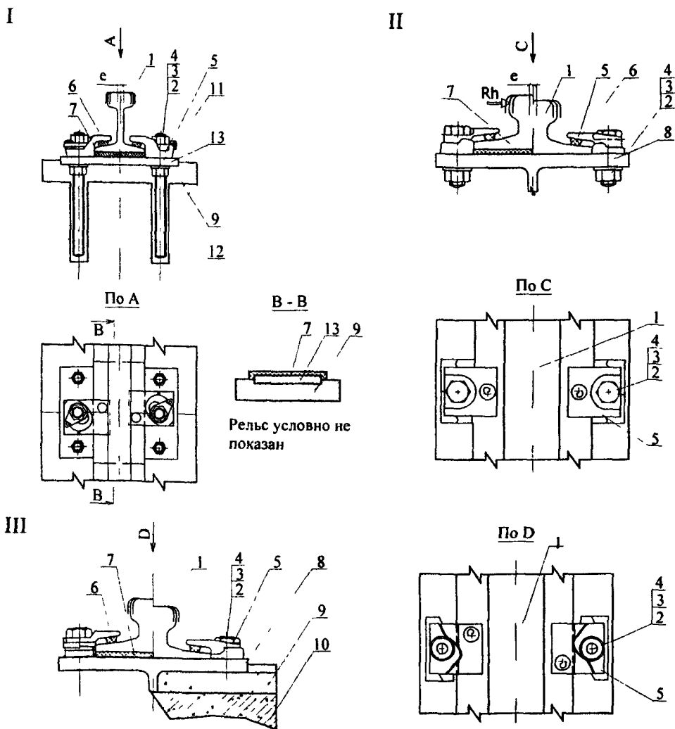
Рис.П.5.11. Промежуточные крепления с эластичным элементом (типа GANTREX):
