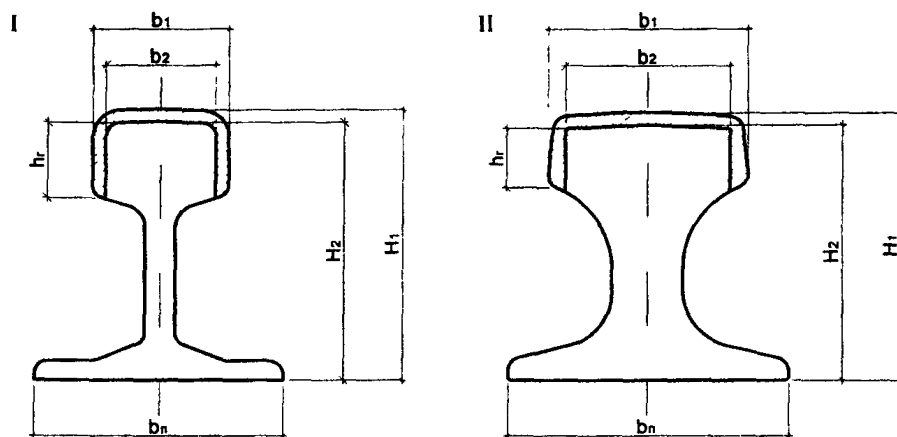
Рис.П.5.1. Поперечный профиль направляющих
