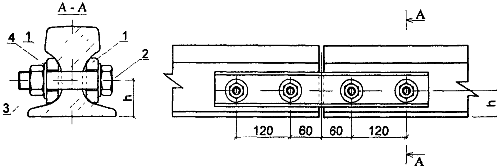
Рис. П.5.4. Разъемное стыковое скрепление для направляющих типа КР.
