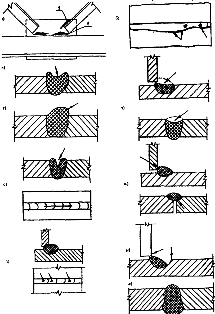
Рис. П.7.1. Дефекты и повреждения сварных соединений стальных элементов и конструкций кранового пути.
