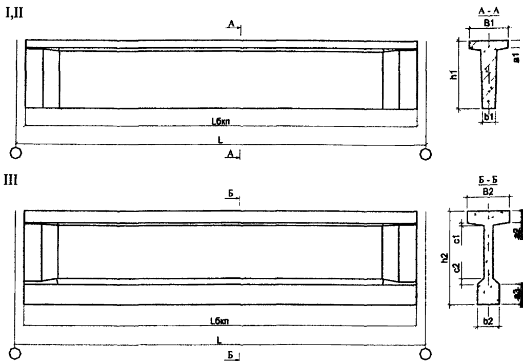
Рис. П.5.16. Типовые конструкции железобетонных балок надземных крановых путей.
