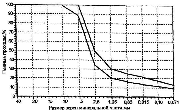
Рисунок 2. Зерновой состав минеральной части щебнемастичного асфальтобетона типа SMA 6 на битумнорезиновом композиционном вяжущем.
