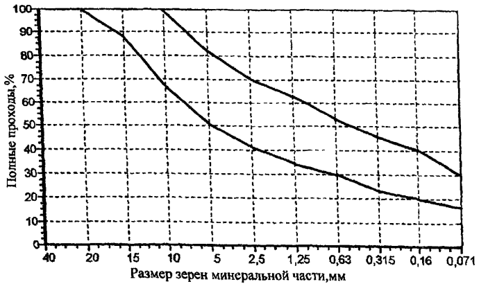
Рисунок 3. Зерновой состав минеральной части асфальтобетона литого типа на битумнорезиновом композиционном вяжущем для механизированной технологии укладки.
