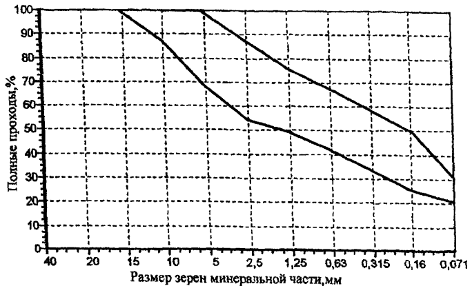
Рисунок 4. Зерновой состав минеральной части асфальтобетона литого типа на битумнорезиновом композиционном вяжущем для ручной технологии укладки.
