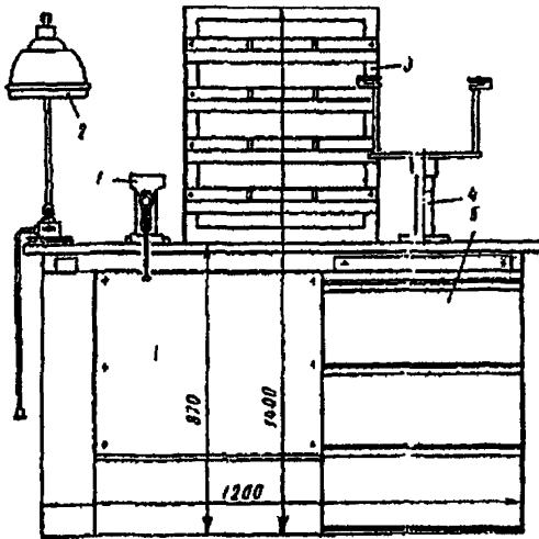
Рис. 5.9. Пост Р-991 текущего ремонта ГА:
