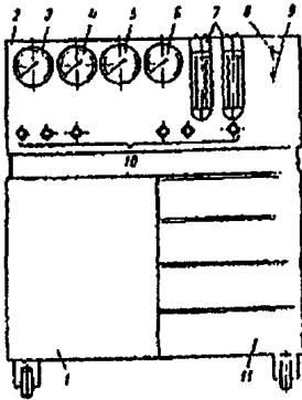
Рис. 5.7. Передвижная установка К-277 для проверки газовой аппаратуры автомобилей:
