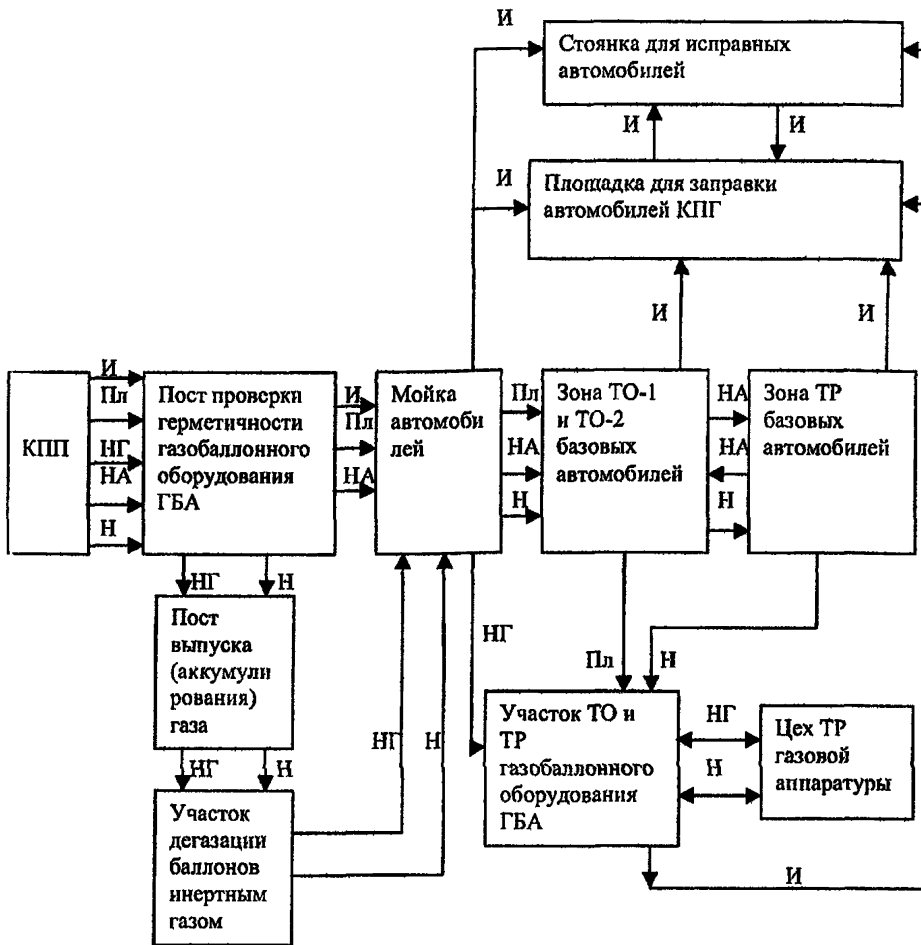
Рис. 5.1. Типовая технологическая схема проведения ТО и ТР газобаллонных автомобилей в условиях АТП:
