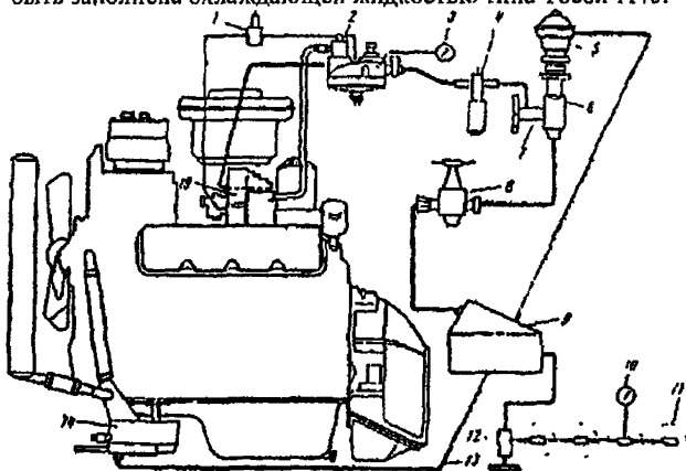
Рис. 7.1. Схема инфраструктуры автономного подогревателя.
