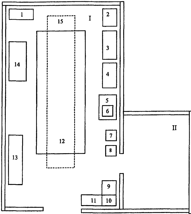
Рис. 5.5. Участок ТО и ТР газобаллонных автомобилей.
