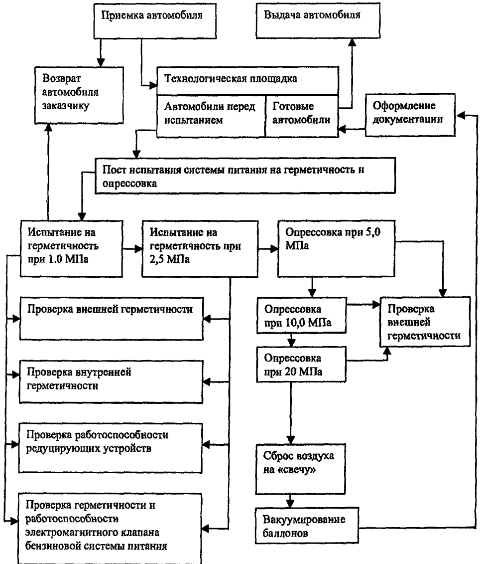
Рис. 9.1. Технологическая схема испытаний автомобилей, работающих на КПП.
