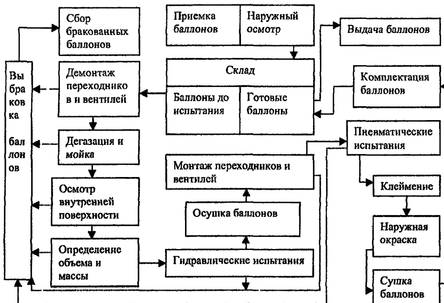
Рис.10.2. Технологическая схема освидетельствования баллонов. Основной маршрут —→ Выбраковка —→
