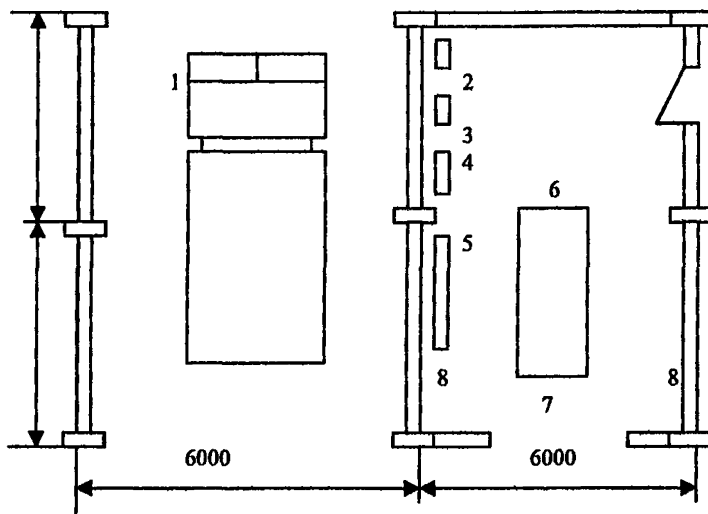
Рис. 5.3. Планировка поста выпуска и аккумуляции газа и дегазации баллонов: 1-бокс для газобаллонных автомобилей на КПГ; 2-пульт управления; 3-кассета баллонов с инертным газом; 4-секция баллонов высокого давления; 5-секция среднего давления; 6-секция низкого давления; 7-бокс для баллонов высокого и низкого давления; 8-перегородка между боксами.
