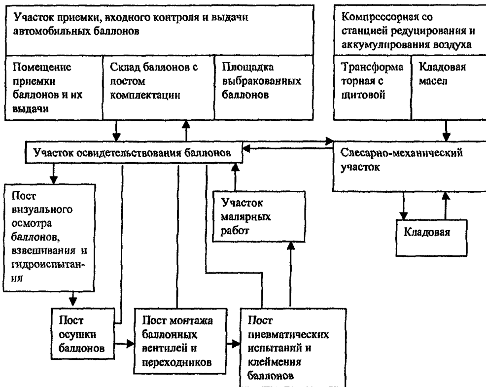
Рис.10.1. Схема пункта освидетельствования баллонов.
